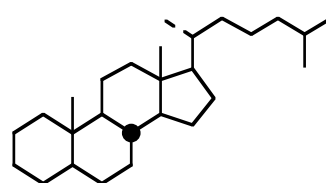
Stéran (C 29 )
