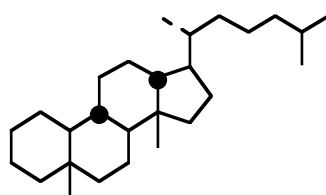
Diastéran (C 29 )
