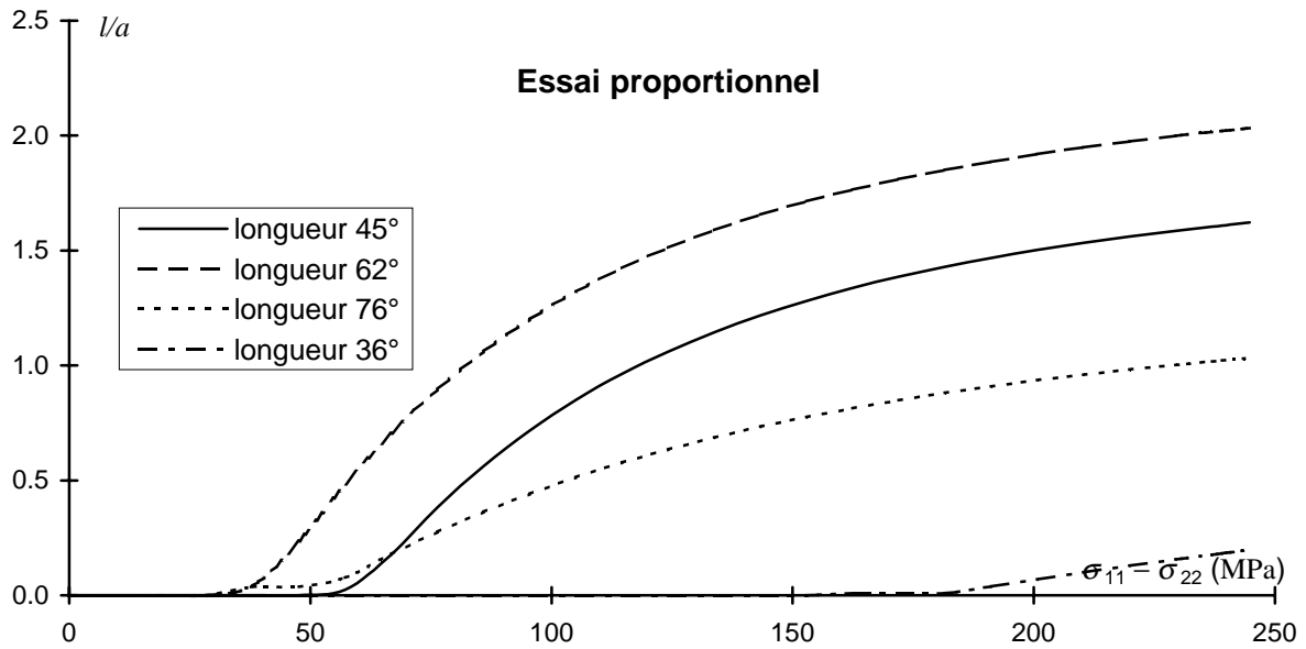
Figure IV.29 : Essai proportionnel : variation des longueurs de branchement.
