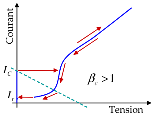
FIG. 1.13. Caractéristique I(V) d'une jonction hystéretique SIS.
