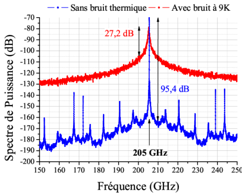
FIG. 3.12. Estimation du spectre de l'horloge en considérant l'influence des fluctuations thermiques à 9K..
