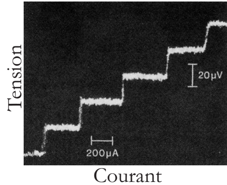
FIG. 1.19. Caractéristique [52] avec éclairage RF (10 GHz) d'une jonction Josephson. La distance entre deux marches est 20,7 \mu\text{V}
