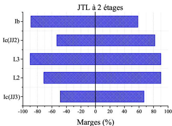
FIG. 3.10. Marges de fonctionnement des jonctions, des inductances et du courant de polarisation de la JTL à deux étages à 205 GHz.
