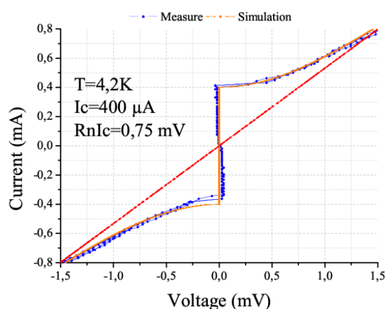
FIG. 4.17. Caractéristique I(V) d'une jonction Josephson de 4 µm de diamètre du procédé SNEP à 5 niveaux pour le jeu de masque SUPRAMOD
