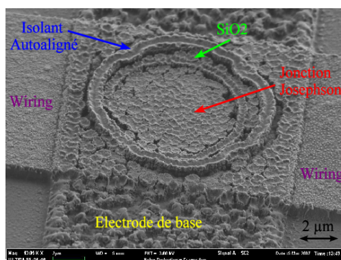
FIG. 4.11. Vue agrandie réalisée au M.E.B. sur la jonction de la figure 4.10.
