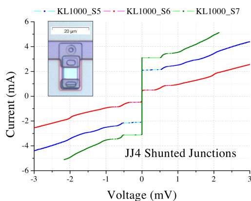
FIG. 5.10. Caractéristique I(V) de la jonction JJ4 avec sa résistance de shunt mesurée sur plusieurs puces (fonderie HYPRES Nb).
