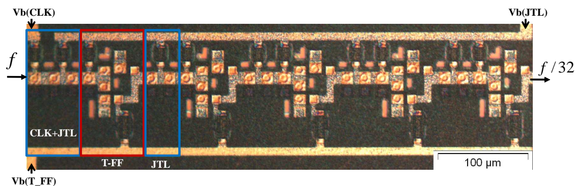
FIG. 4.7. Photographie du diviseur de fréquence (procédé complet à 10 niveaux).
