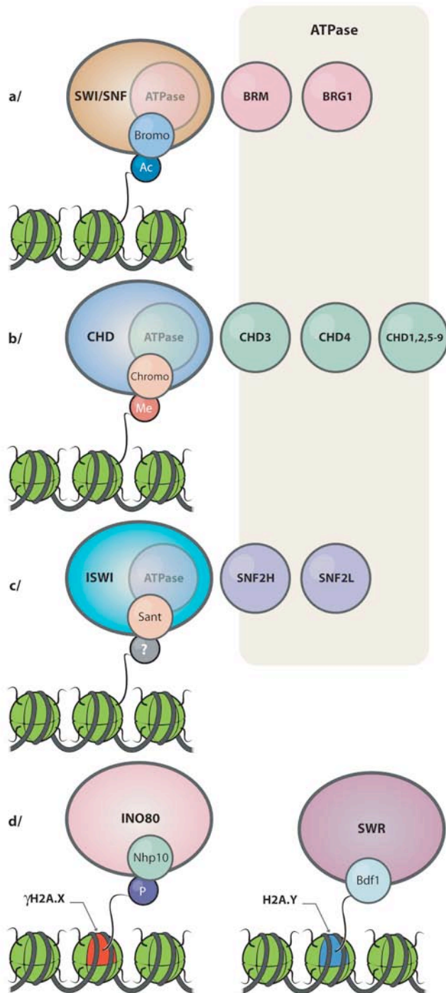
Figure 7 : Facteurs de remodelage de la chromatine ATP-dépendant
