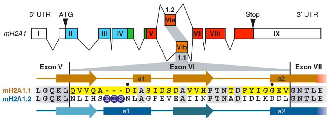
Figure 14 : Epissage alternatif de l'ARNm codant pour macroH2A1.1 et macroH2A1.2
