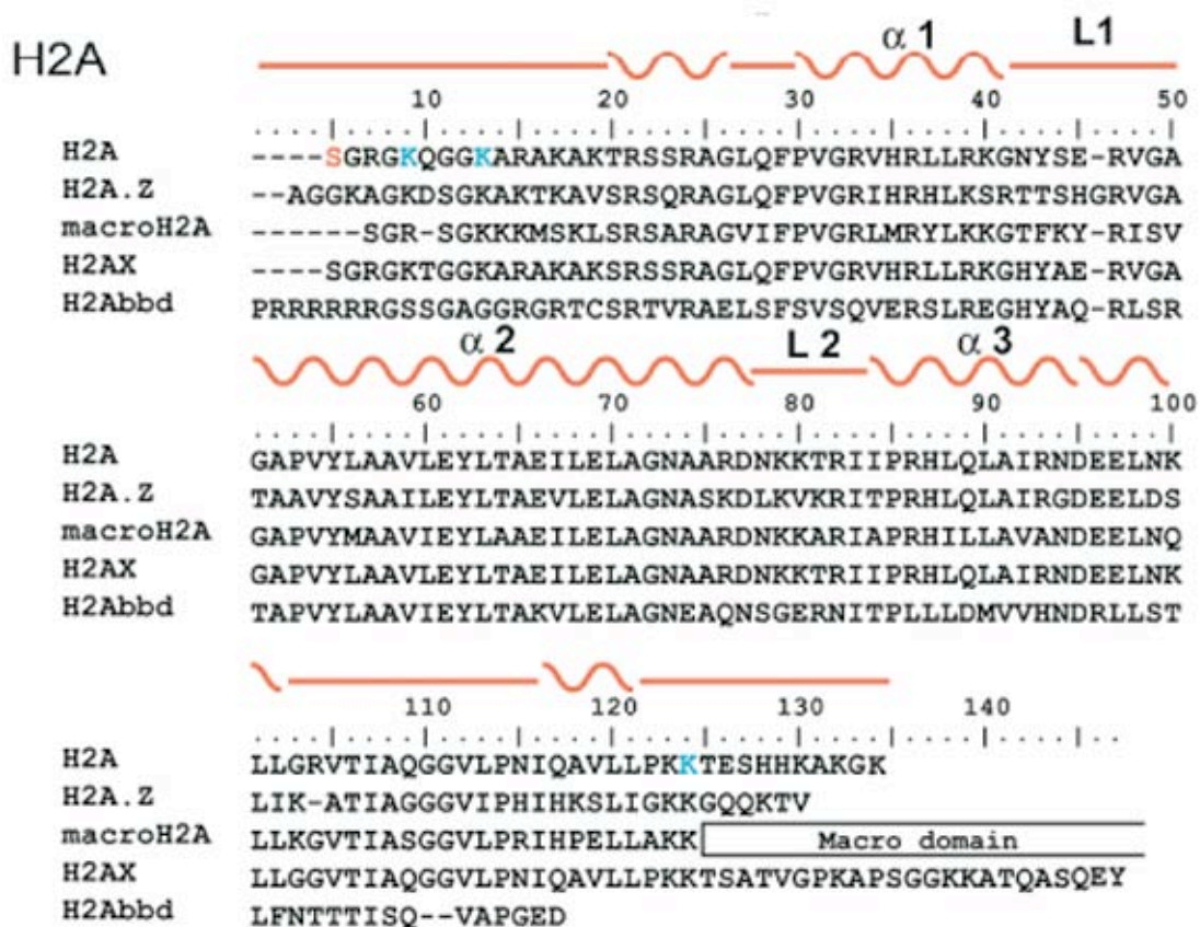
Figure 11 : Alignements de séquences des variants de l'histone H2A
