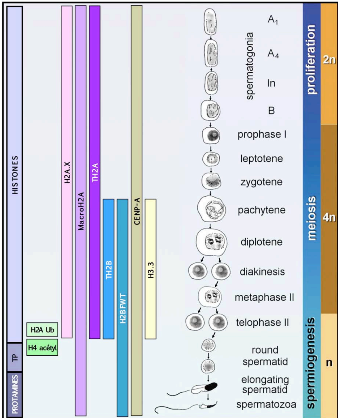
Figure 18 : Composants de la chromatine au cours de la spermatogénèse
