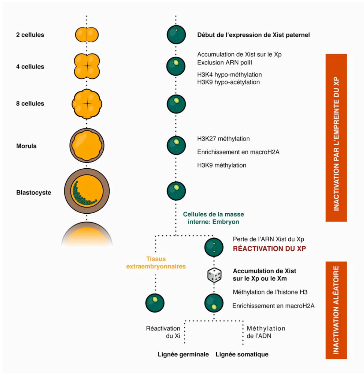
Figure 8 : Cinétique de l'inactivation du chromosome X chez la souris
