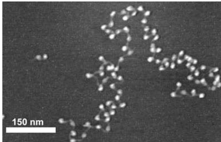
Figure 4 : Image du nucléofilament réalisée par cryo-AFM
