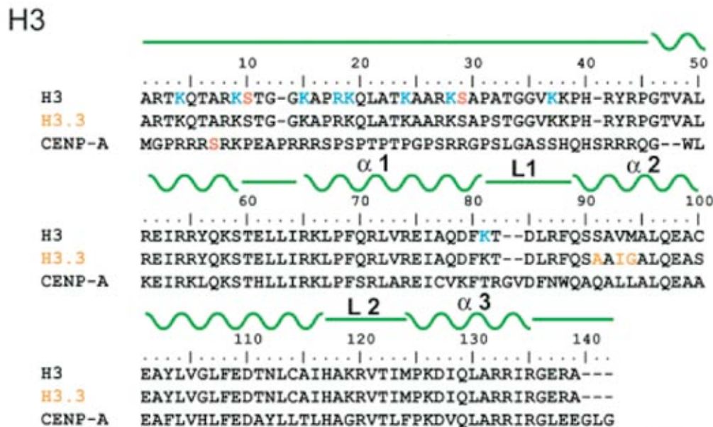
Figure 10 : Alignements de séquences des variants de l'histone H3
