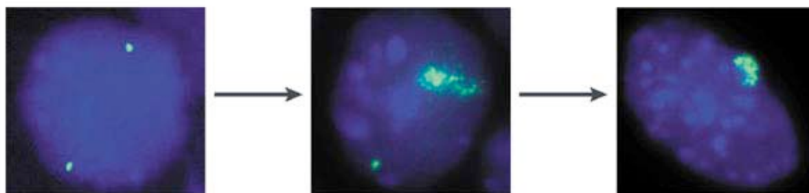
Figure 9 : Expression de l'ARN Xist dans les cellules souches embryonnaires
