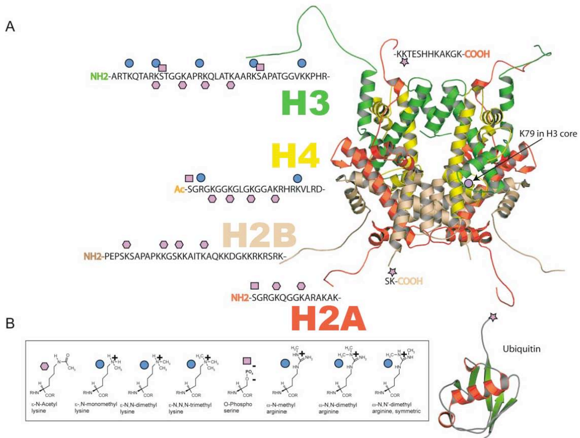
Figure 17 : Représentation des principales modifications post-transcriptionnelles des histones
