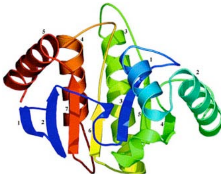
Figure 13 : Structure cristallographique du domaine macro AF1521
