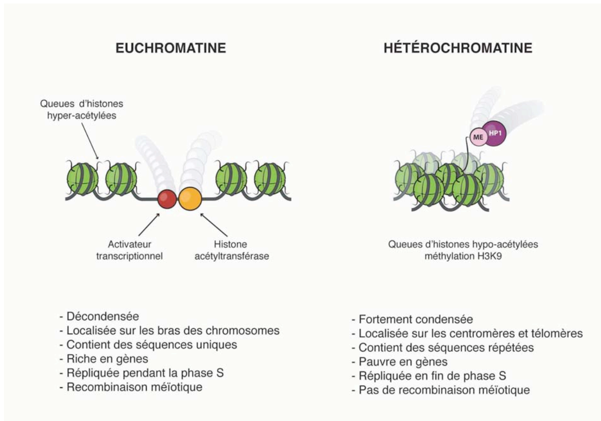
Figure 5 : Propriétés des régions euchromatiques et hétérochromatiques
