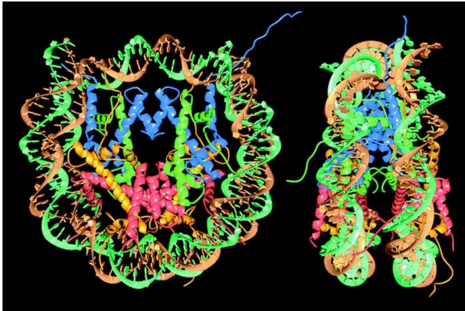
Figure 1 : Structure cristallographique du nucléosome à 2,8 Å
