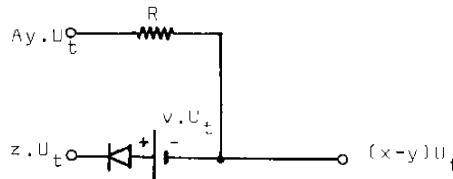
Figure 4.8. : Atténuateur variable
