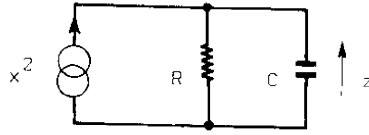
Figure 4.5. : Redresseur quadratique
