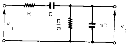
Figure 4.2 : Déphaseur de Wien
