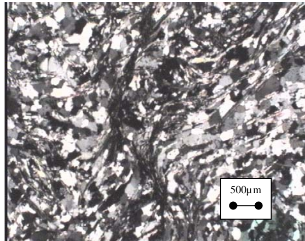
Figure 4.5c et d. Métapélite 04SJ6. deux types de microplissements formés par les phengites, marquant deux schistosités.
