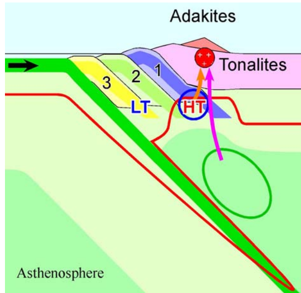
Figure 6.4b. Formation des intrusifs adakitiques
