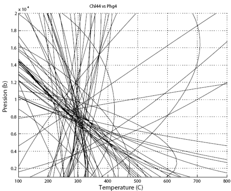
Figure 4.18c. Résultats obtenus par la méthode des multi-équilibres sur les couples en haut : chl 44 - phg 2 en bas : chl 44 - phg 4.
