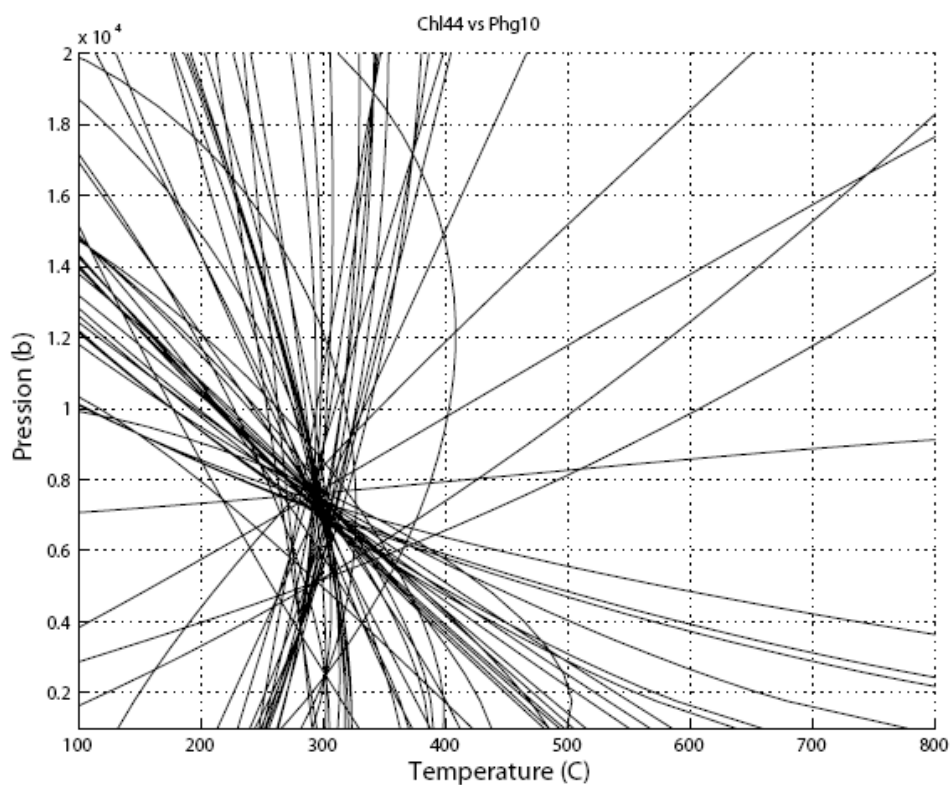
Figure 4.18b. Résultats obtenus par la méthode des multi-équilibres sur les couples chl 44 - phg 10.
