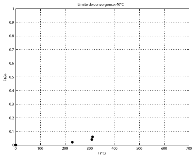
Figure 4.15. Proportion de Fe^{3+} / Fe_{tot} estimée pour chaque chloritoïde en 04SJ6, afin d'avoir cristallisation à P=7kb , pour des températures de cristallisation variables.
