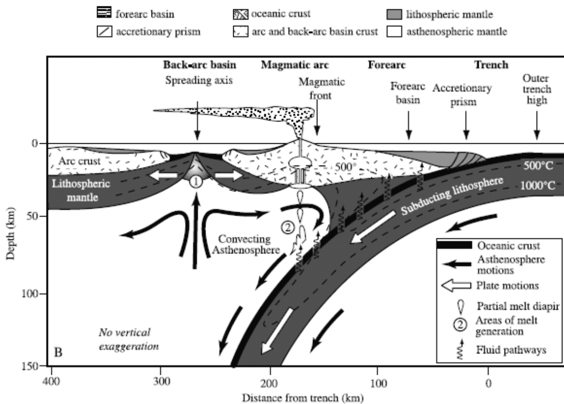
Figure 1.1a. Profil de la subduction d'une plaque océanique sous une lithosphère continentale (d'après Stern, 2002). Voir aussi figure 1.2a
