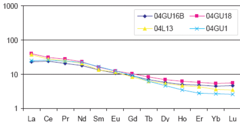
Figure 5.23a. REE des microdiorites, normalisés par rapport aux chondrites (Sun and McDonough, 1989).
