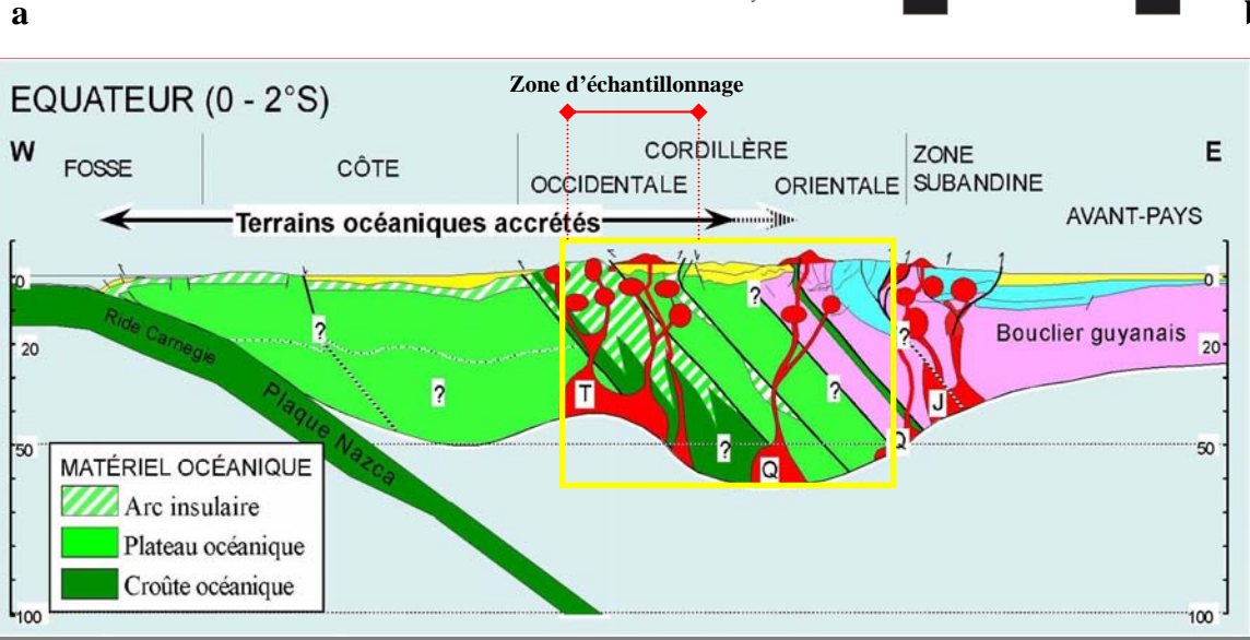
Figure 1.21. Coupe schématique de l'Equateur. Les terrains océaniques accrétés pendant au Crétacé supérieur à Paléogène à la marge W de l'Equateur et qui constituent actuellement la racine crustale des Andes. Noter les intrusions néogènes liées à l'arc volcanique (d'après Jaillard, 2002).
