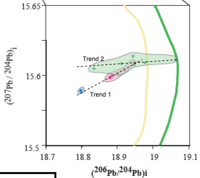
Figure 5.28a (en haut) Diagramme (^{207}\text{Pb}/^{204}\text{Pb})_i vs (^{206}\text{Pb}/^{204}\text{Pb})_i , les intrusifs miocène tombent dans la zone des OIB et la zone des adakites récents (Bourdon et al., 2003) sauf le microgabbro 04L18 qui se situe dans la zone des roches d'arc magmatique d'âge Miocène à récent (Chiaradia et al., 2004).
