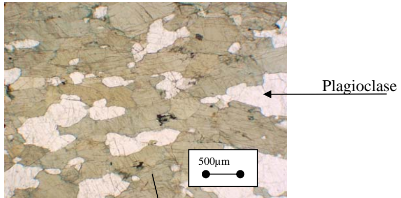
Figure 4.3. Métagabbro (04GU12). Composition des amphiboles (Nomenclature d'après Leake et al., 1997) et des plagioclases
