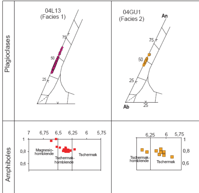
Figure 5.12. Composition chimique des minéraux des microdiorites de faciès 1 et 2
