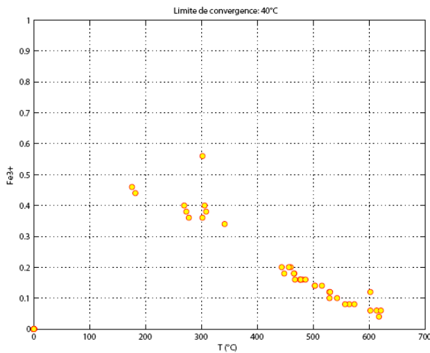
Figure 4.14. Proportion de Fe^{3+} / Fe_{tot} estimée pour chaque chlorite en 04SJ1, afin d'avoir cristallisation à P=7kb , pour des températures de cristallisation variables.
