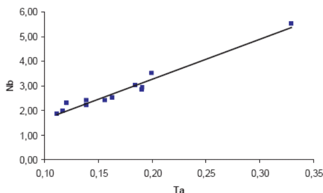
Figure 5.18. Diagramme de corrélation entre les couples d'éléments Zr vs Hf et Nb vs Ta. L'excellente corrélation observée indique que ces éléments n'ont pas été remobilisés durant l'altération.
