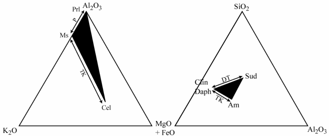
Figure 4.8. A droite , diagramme ternaires Al-K-(Fe+Mg) pour les micas A gauche : Si-Al-(Fe+Mg) pour les chlorites, et les trois substitutions principales : Tschermak (TK), Pyrophyllitic (P) et Di/Trioctahédrale (DT).
