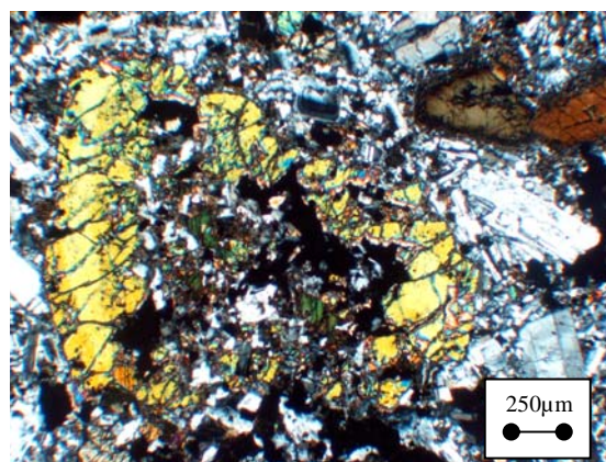
Figure 5.8b. Microgabbro à amphibole, 04L17. Plagioclases, clinopyroxènes et amphiboles brunes altérés
