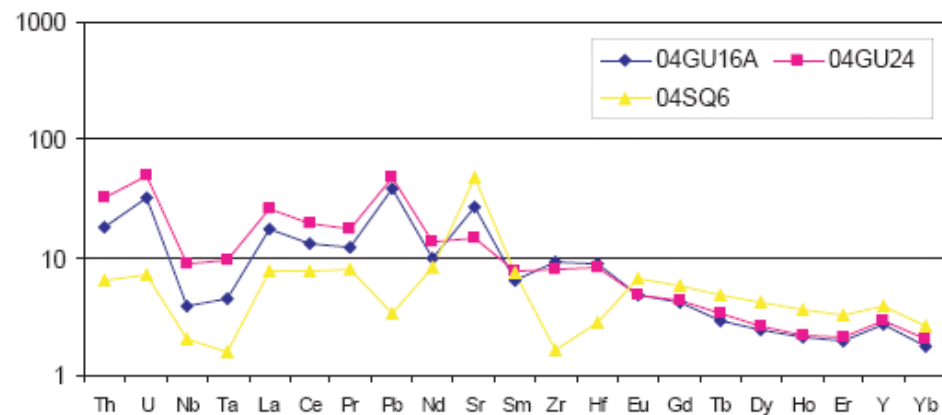
Figure 5.24b. Éléments traces des dacites et de la monzodiorite 04SQ6, normalisés par rapport au manteau primitif (Sun and McDonough, 1989).
