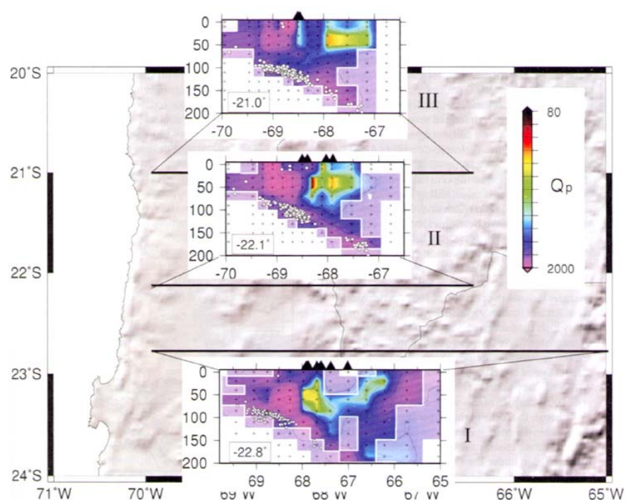
Figure 6.3a. Profils tomographiques E-W des Andes du centre-nord du Chili. Ces modèles montrent une atténuation sismique (en jaune et rouge) en profondeur, suggérant la présence de «liquides» issus de la fusion partielle de la croûte inférieure (Schilling et al., 2006).
