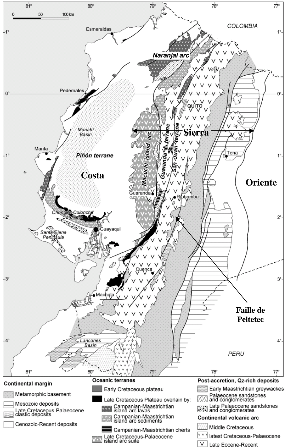
Figure 1.14. Terrains océaniques accrés à la marge W de l'Equateur, (D'après, Jaillard et al., 2002).
