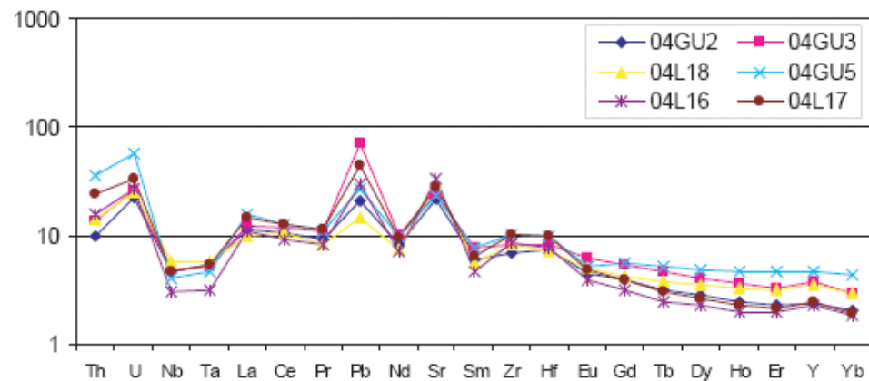
Figure 5.22b. Éléments traces des microgabbros, normalisés par rapport au manteau primitif (Sun and McDonough, 1989).
