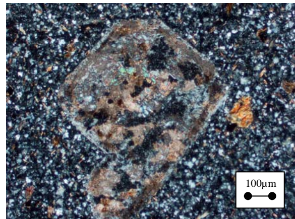
Figure 5.13b. Dacites de faciès 1, 04GU16A. Plagioclase calcitisé.
