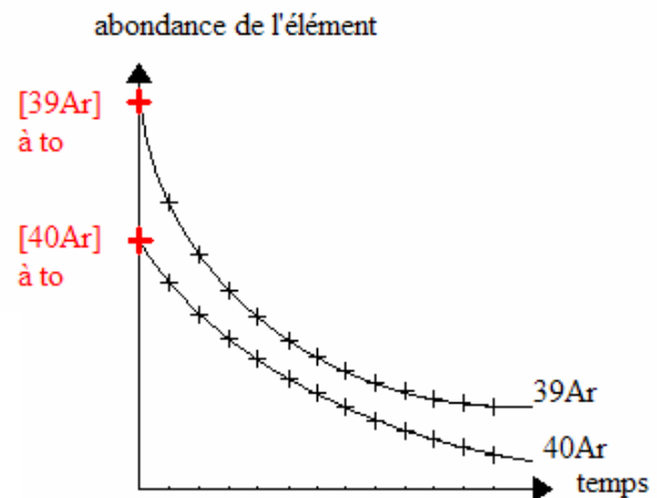
Figure 2.8. Graphe théorique de l'abondance, de deux des éléments mesurés par le spectromètre, en fonction du temps. Le calcul du rapport ^{40}\text{Ar}/^{39}\text{Ar} au temps « t_0 » permet de trouver l'âge apparent du palier de température.
