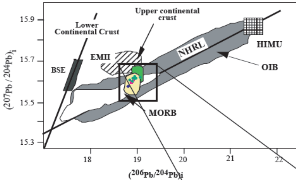
Figure 5.28a (en haut) Diagramme (^{207}\text{Pb}/^{204}\text{Pb})_i vs (^{206}\text{Pb}/^{204}\text{Pb})_i , les intrusifs miocène tombent dans la zone des OIB et la zone des adakites récents (Bourdon et al., 2003) sauf le microgabbro 04L18 qui se situe dans la zone des roches d'arc magmatique d'âge Miocène à récent (Chiaradia et al., 2004).
