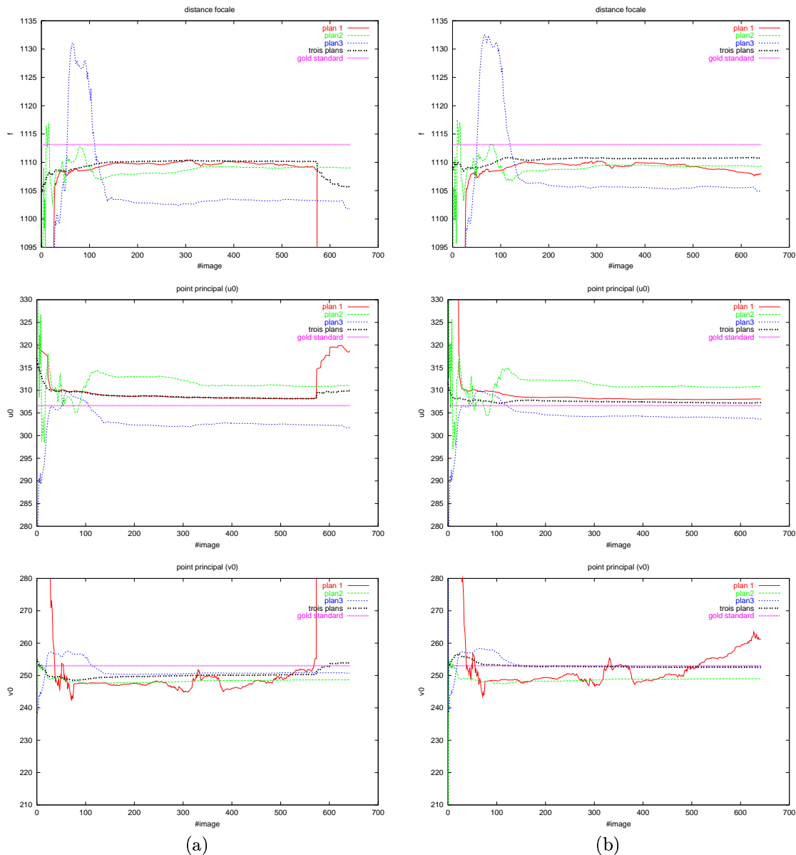
FIG. 7.10 – Méthode de Sturm-Maybank : paramètres intrinsèques calculés (f, u_0, v_0) , lorsque \tau est connu ; pour les cas planaire et multiplanaire, (a) à partir de la méthode originale et (b) avec l'intégration de la technique de pondération statistique.
