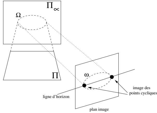
FIG. 6.3 – La conique absolue, les points cycliques, et leurs images correspondantes.
