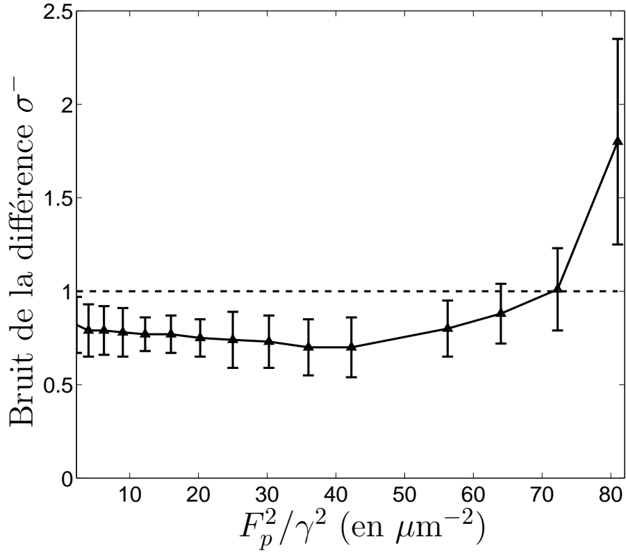
FIG. 3.16: Résultat du calcul de Monte Carlo Quantique sur le bruit de la différence en intensité des modes du signal et du complémentaire \sigma^- en fonction de la puissance de pompe dans un potentiel désordonné. La ligne reliant les points du graphique est un guide pour l'oeil. Les barres d'erreurs correspondent à l'écart type de la moyenne en fonction du temps une fois le régime stationnaire atteint. Les paramètres utilisés sont les même que pour la figure 3.4.
