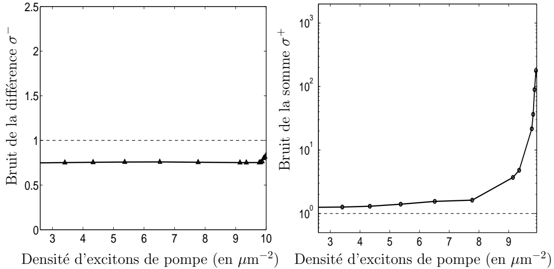
FIG. 3.20: Bruit de la somme (à droite) et de la différence (à gauche) en intensité des faisceaux du signal et du complémentaire en fonction de la densité d'excitons dans de pompe, calculé par l'intermédiaire du modèle analytique, dans un potentiel non désordonné, avec un état d'entrée vide. Les paramètres utilisés sont les même que pour la figure 3.19.
