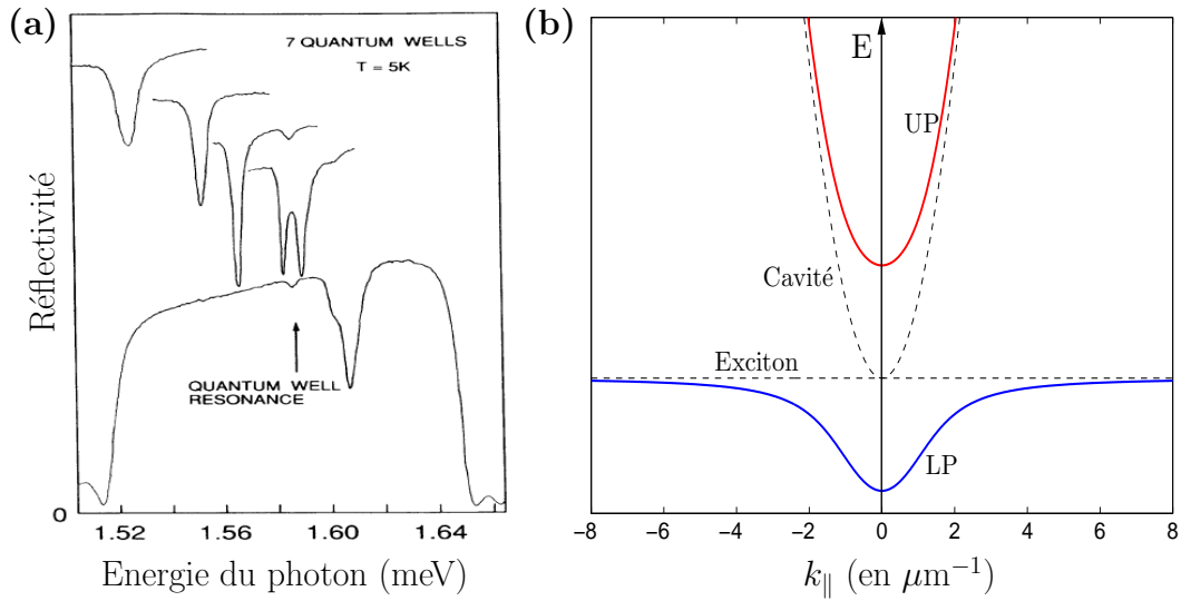
FIG. 1.9: (a) Spectres de réflectivité obtenus à 5K pour différents désaccords entre la cavité et le puits quantique [3]. (b) Courbes de dispersion des polaritons (lignes continues), et de l'exciton et du photon (traits pointillés).
