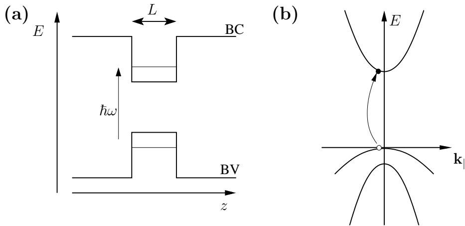
FIG. 1.1: (a) Niveaux d'énergie dans un puits quantique et transition interbande entre les bandes de valence (BV) et de conduction (BC) correspondantes. (b) Dispersion des bandes et processus de création d'une paire électron-trou correspondant.
