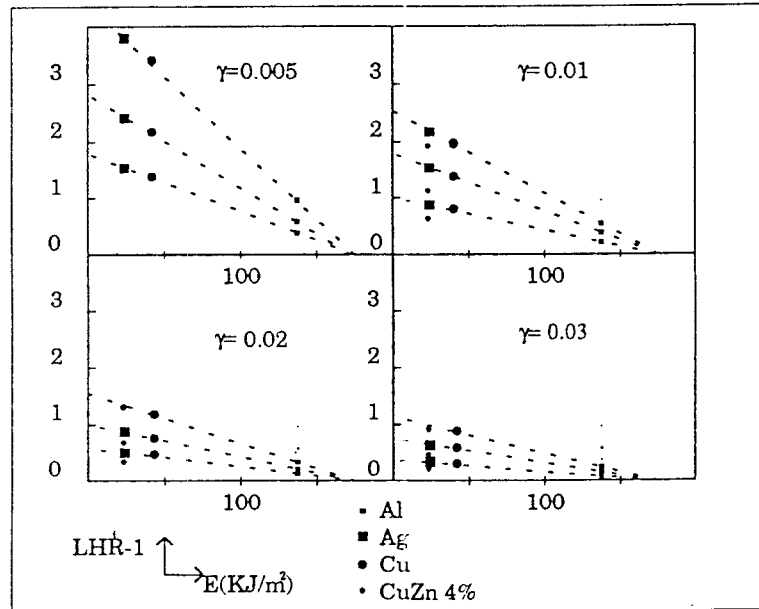
Figure 1.14: Variation de l'anisotropie de l'écaouissage en fonction de l'énergie de faute d'empilement E et pour diverses valeurs du glissement primaire. [Fra84]
