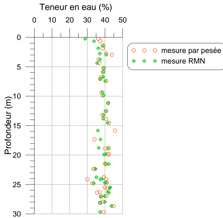
Figure 2-28. Profil des teneurs en eau sur un forage de Warloy-Baillon
