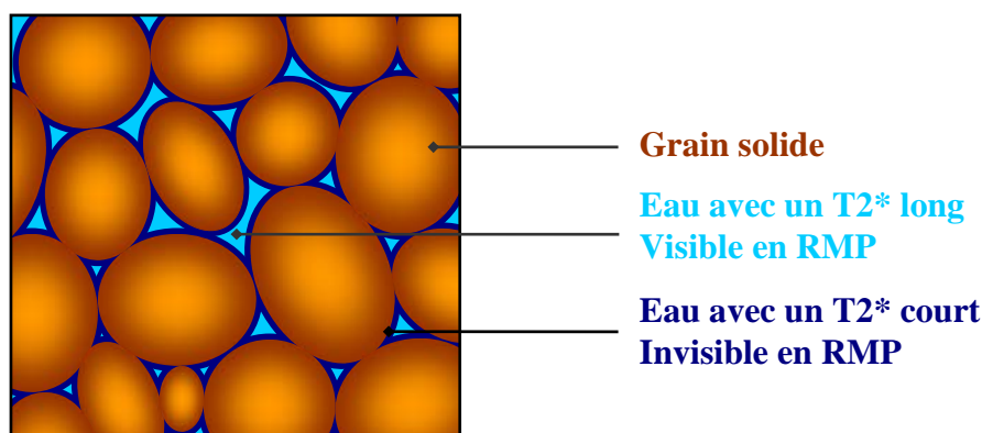
Figure 1-34. Déteçtabilité de l'eau en RMP
