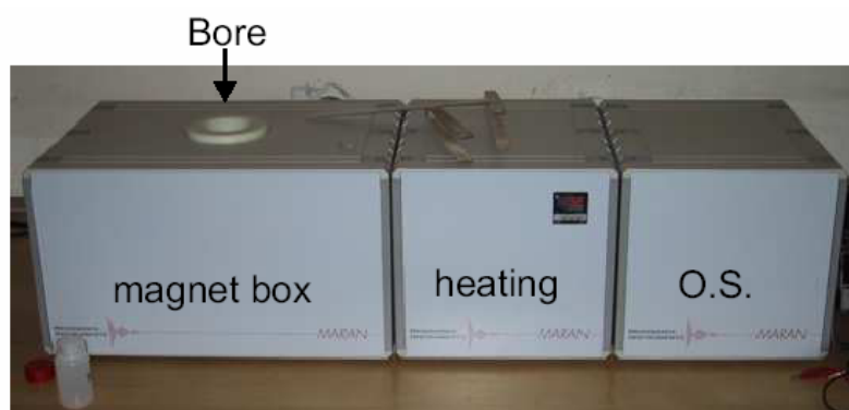
Figure 1-18. Spectromètre RMN Maran Ultra 2 MHz
