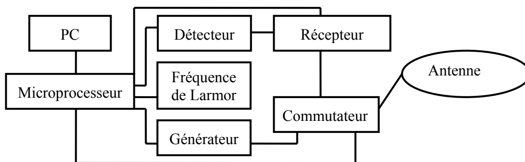
Figure 1-28. Schéma fonctionnel du dispositif instrumental NUMIS
