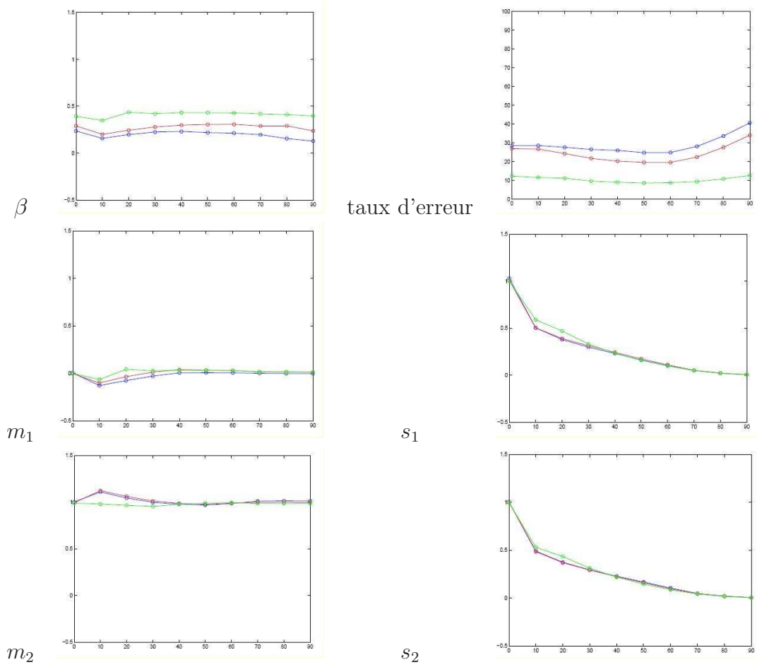
Fig. 5.16: Estimation des paramètres du modèle et taux de classification pour les trois simulations de 5.7 : \beta = 0, 2 (bleu), 0, 3 (rouge) et 0, 4 (vert) dans le cas où la totalité des données manquantes sont NMAR censurées à gauche et à droite ( \sigma^2 = 1 ).
