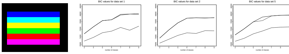
Fig. 5.2: Classification de référence et courbes BIC pour trois jeux de données lorsque K varie de 3 à 9. La ligne pleine est celle correspondant à l'algorithme en champ simulé tandis que la ligne pointillée est celle de l'algorithme EM standard et la ligne interrompue celle de l'algorithme en champ moyen.
