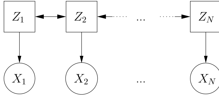
Fig. 3.4: Chaîne de Markov cachée bilatérale (ou non causale)
