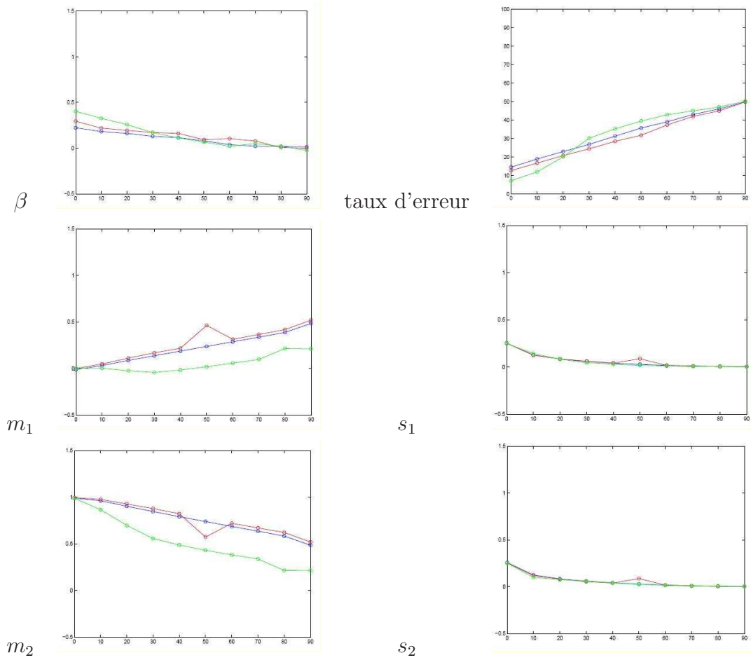
Fig. 5.14: Estimation des paramètres du modèle et taux de classification pour les trois simulations de 5.7 : \beta = 0,2 (bleu), 0,3 (rouge) et 0,4 (vert) dans le cas où la totalité des données manquantes sont NMAR censurées à gauche et à droite ( \sigma^2 = 0,25 ).
