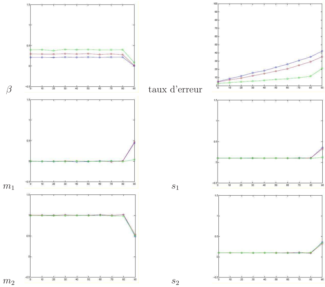
Fig. 5.10: Estimation des paramètres du modèle et taux de classification pour les trois simulations de 5.7 : \beta = 0, 2 (bleu), 0, 3 (rouge) et 0, 4 (vert) dans le cas où les données manquantes sont MCAR ( \sigma^2 = 0, 1 ).
