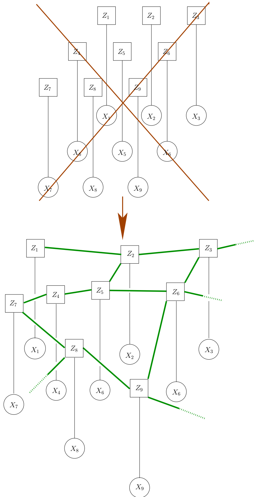
Fig. 3.5: Graphe de champ de Markov caché (en bas) par opposition au modèle de mélange sur le même champ (en haut).
