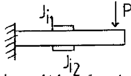
FIGURE IV.8 Disposition des jauges sur une poutre
