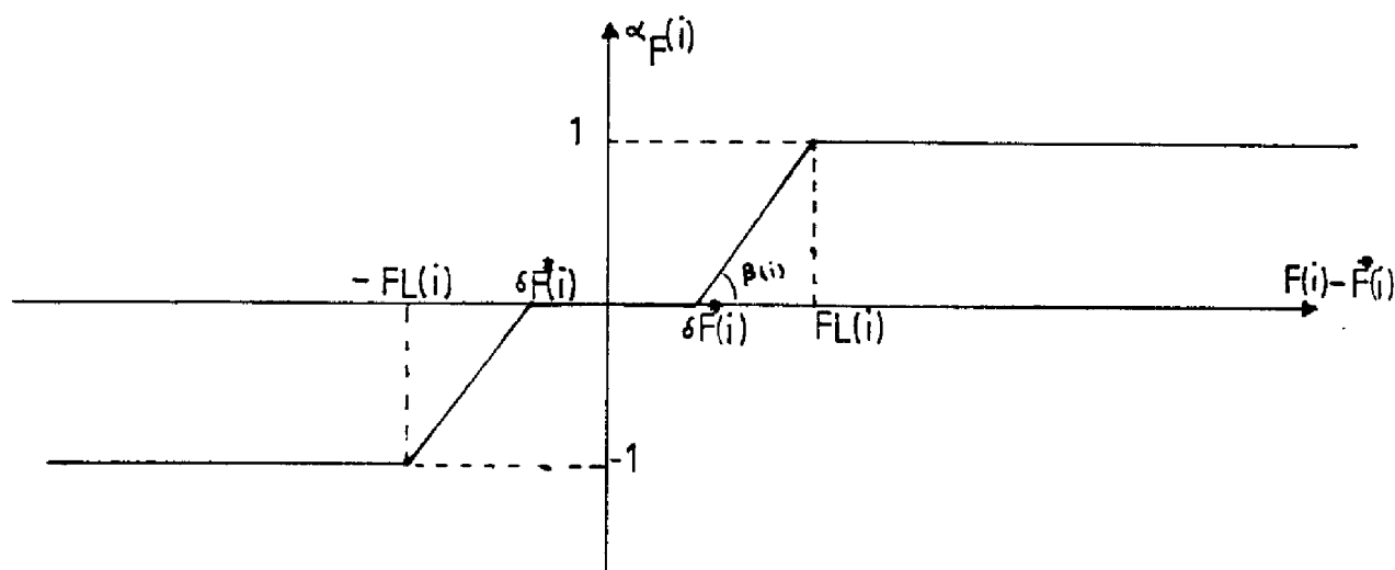
FIGURE III.9 Fonction réalisant l'asservissement en force
