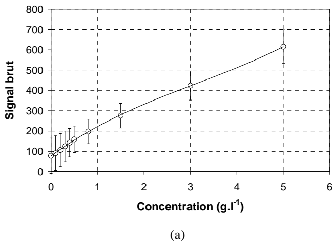
Figure 88 : (a) courbe d'étalonnage moyenne de l'ASM-IV Argus à partir des sédiments de la Vilaine (la variabilité est déterminée à partir des moyennes des 144 capteurs) ; (b) dispositif d'étalonnage : perche placée dans un tube PVC et circulation (de haut en bas) du fluide (eau + sédiments) assurée par une pompe. La partie basse du tube est conique pour éviter les zones locales de dépôt et l'ensemble est protégé de la luminosité ambiante.
