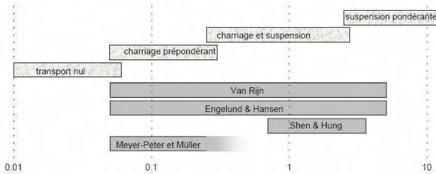
Figure 62 : Validité de différentes formules de transport solide en fonction du régime de transport caractérisé
