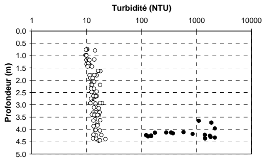
Figure 79 : Turbidités mesurées au pont du Grand Pas le 12/04/2005, à 30 m de la rive gauche, lors de la descente de la sonde (○), puis de sa remontée (●).
