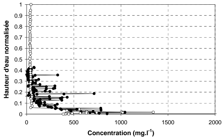
Figure 91 : Exemple de superposition de profils de concentration non instantané (o) et instantané (●) en amont du pont du Grand Pas.
