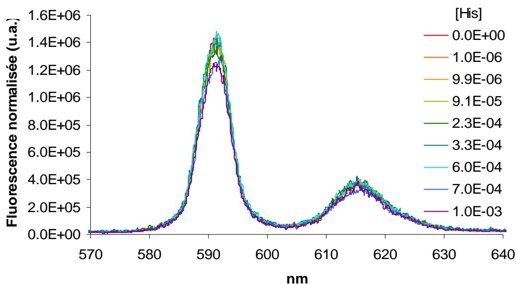
Figure 52 : Dosage Eu (10 -6 M)-Histidine (de 0 à 0,001 M) à pH 3 par SLRT ( E_{exc} = 395,2 \text{ nm} ; E_{laser} = 0,7 \text{ mJ} ; D = 1 \text{ }\mu\text{s} ; L = 500 \text{ }\mu\text{s} )
