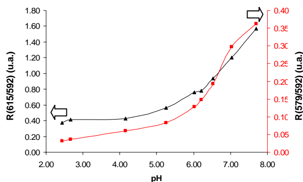
Figure 54 : Evolution des rapports des intensités de fluorescence (Eu+His=f(pH))
