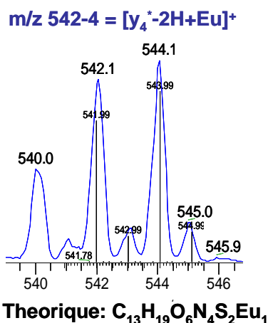
Figure 106 : Identification du complexe
