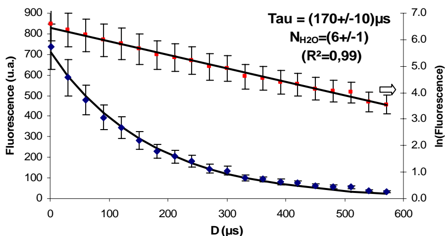
Figure 56 : Evaluation du temps de vie du complexe Eu (10 -6 M) + Histidine (0,05M) pH 7,7
