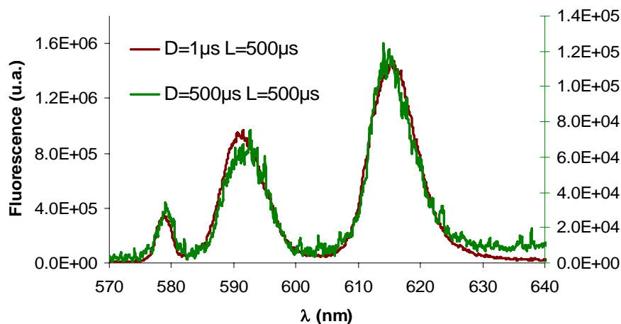
Figure 55 : Comparaison des spectres mesurés pour D=1 \mu s et D=500 \mu s sur une solution Eu (10 -6 M) + Histidine (0,05M) pH 7,7 ( \lambda_{exc} = 395,2 nm ; E~0,7mJ ; L=500 \mu s)
