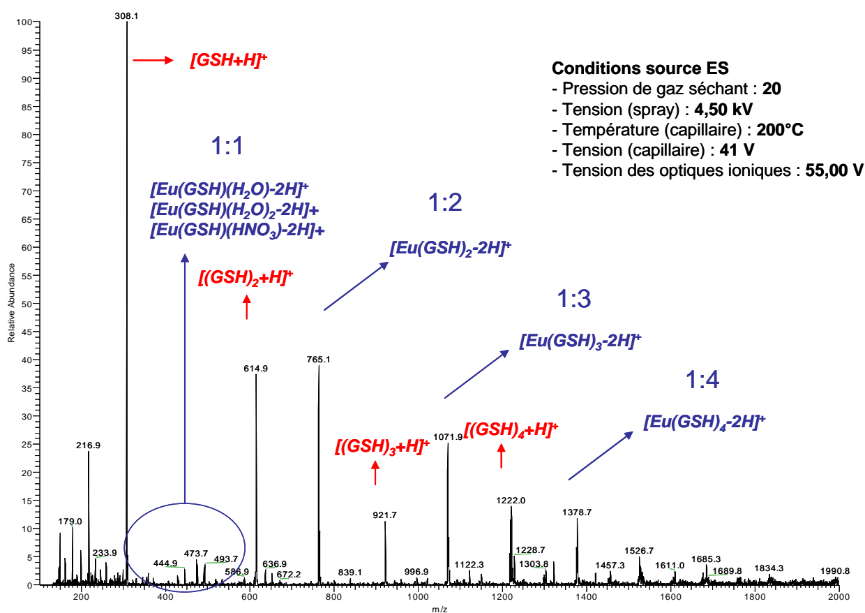
Figure 68 : Spectre de masse : \text{Eu}(\text{NO}_3)_3 10^{-4}\text{M} + GSH 10^{-3}\text{M} ( \tau = 10 ) pH 3,0 ; Mode ES+
