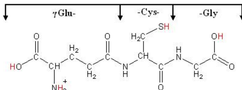
Figure 57 : Molécule de GSH : H 4 L +
