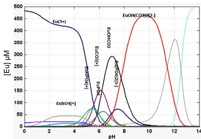
Figure 110 : Diagramme de spéciation de Eu ( [Eu(NO_3)_3]=500\mu M ) dans le milieu de culture des cellules (composition en Annexe 5). Diagramme réalisé avec le logiciel J-CHESS (Van Der Lee et De Windt, 2002), les données thermodynamiques proviennent de la base de données de l'IUPAC (Powell, 2004).
