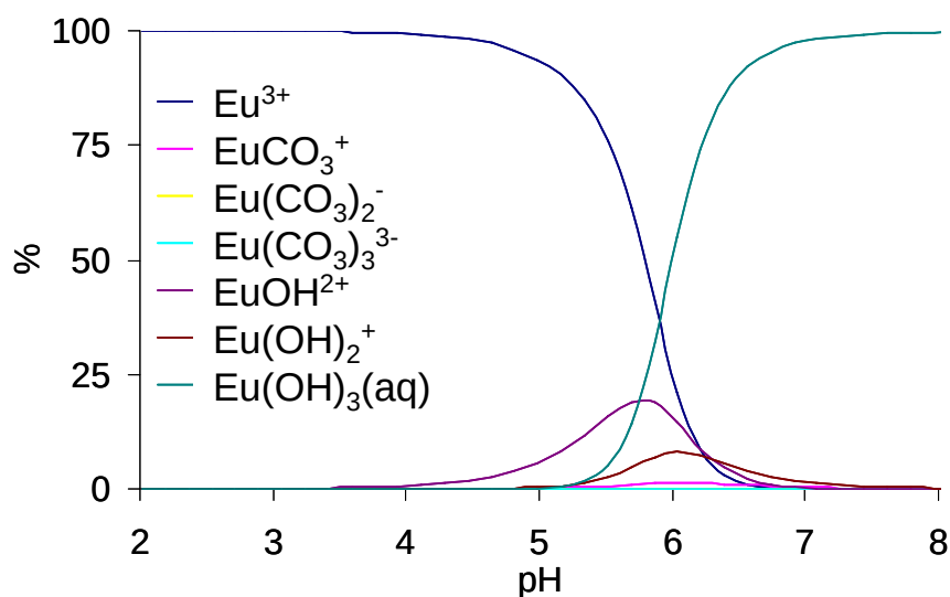
Figure 4 : Diagramme de spéciation de Eu(III) à 10^{-6}\text{M} en fonction du pH ( p_{\text{CO}_2} atmosphérique, 25°C) Les données thermodynamiques proviennent de Nagra/PSI : Chemical Thermodynamic Data Base (Hummel et al. , 2002).
