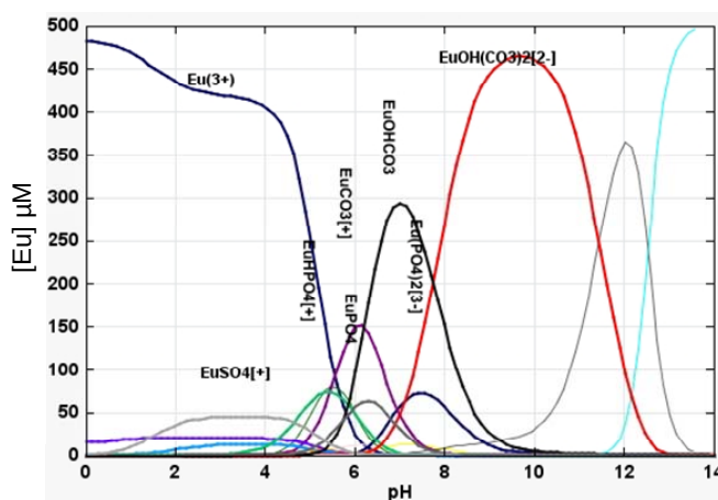
Figure 110 : Diagramme de spéciation de Eu ( [\text{Eu}(\text{NO}_3)_3]=500\mu\text{M} ) dans le milieu de culture des cellules (composition en Annexe 5). Diagramme réalisé avec le logiciel J-CHESS (Van Der Lee et De Windt, 2002), les données thermodynamiques proviennent de la base de données de l'IUPAC (Powell, 2004).
