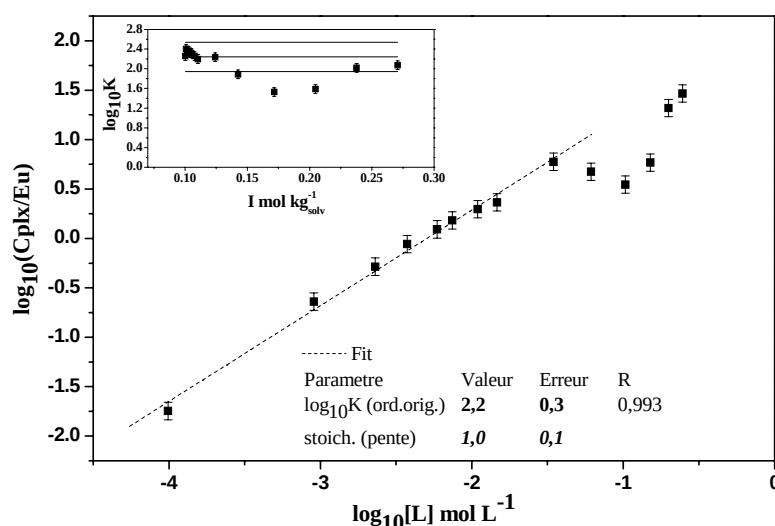
Figure 73 : Stoechiométrie et constante de formation d'un complexe : dosage Eu + GSH pH 6 ( [\text{Eu}] = 10^{-6} \text{ M} )
