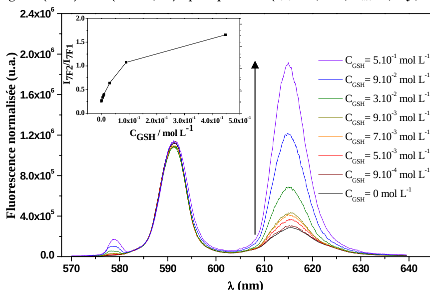
Figure 64 : Dosage Eu ( 10^{-5} M)-GSH (de 0 à 0,5M) à pH 3 par SLRT ( \lambda_{\text{exc}}=395,7\text{nm} ; E_{\text{laser}}=0,9\text{mJ} ; D=1\mu\text{s} ; L=300\mu\text{s} )
