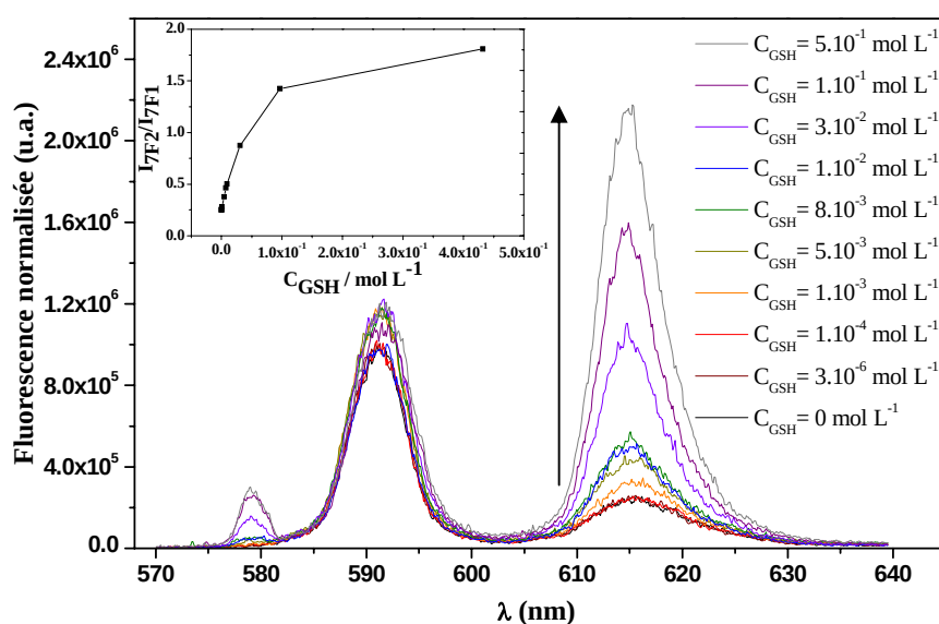
Figure 63 : Dosage Eu ( 10^{-6} M)-GSH (de 0 à 0,5M) à pH 3 par SLRT ( \lambda_{\text{exc}}=395,7\text{nm} ; E_{\text{laser}}=0,9\text{mJ} ; D=1\mu\text{s} ; L=300\mu\text{s} )
