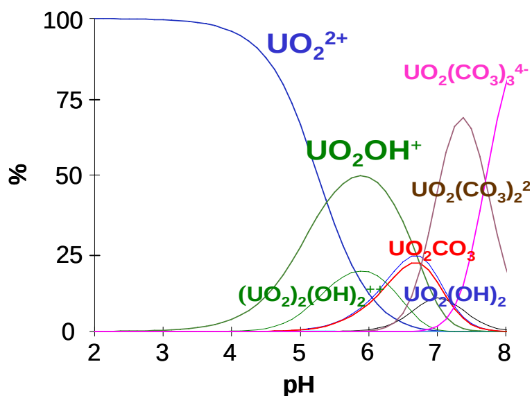
Figure 5 : Diagramme de spéciation de U(VI) à 4.10^{-6}\text{M} en fonction du pH ( p_{\text{CO}_2} atmosphérique, 25°C) Les données thermodynamiques proviennent de NEA-TDB-OECD (Grenthe et al. , 1992) et (Vitorge et Capdevila, 2003).
