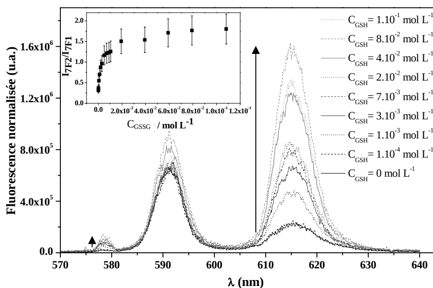
Figure 77 : Dosage Eu (10 -6 M)-GSSG (de 0 à 0,1 M) à pH 6 par SLRT (λ exc = 395,7 nm ; E laser = 0,9 mJ ; D = 1 μs ; L = 500 μs)
