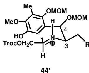
Figure 7. Etat de transition de l'intermédiaire iminium 44' . 39
