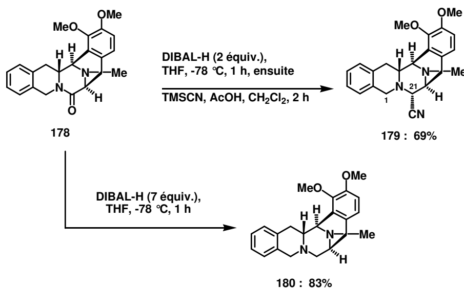
Schéma 40. Synthèse de l' \alpha -amino-nitrile 179 et de la benzylamine 180 .
