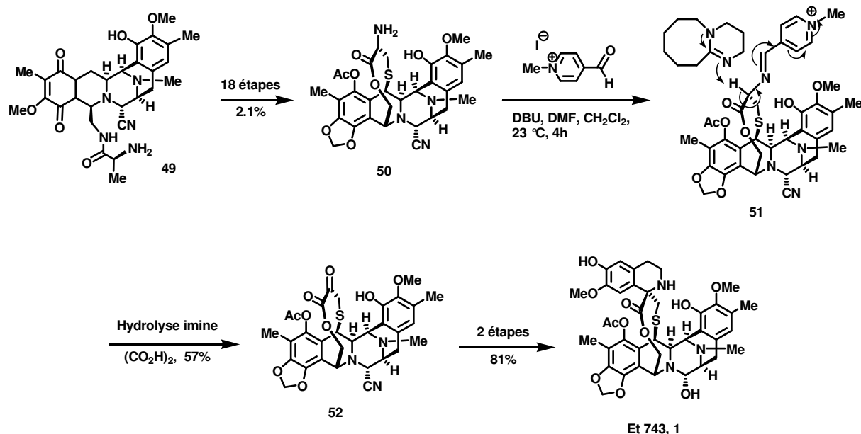
Schéma 6. Hémisynthèse de l'Et 743 à partir de la cyanosafraïne B. 12
