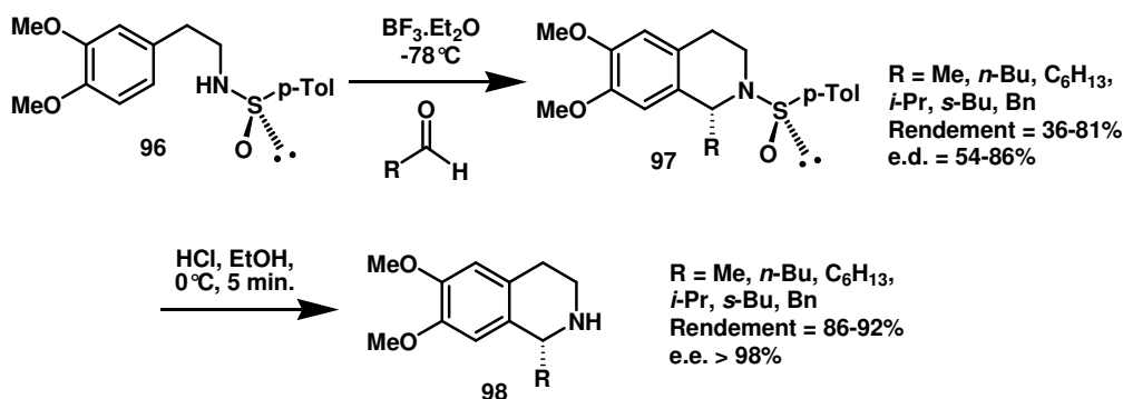
Schéma 15. Synthèse de tétrahydroisoquinoléines énantipures. 62
