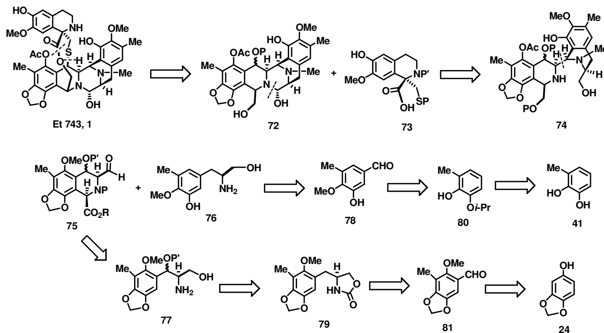
Schéma 10. Schéma rétrosynthétique envisagé pour l'Et 743.
