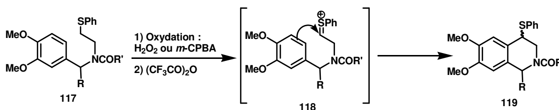
Schéma 20. Cyclisation de Pummerer. 68b
