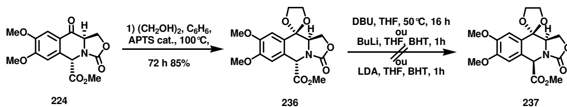
Schéma 55. Tentatives d'épimérisation de 236 en 237 .
