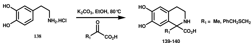
Schéma 27. Cyclisation directe de Pictet-Spengler avec la dopamine. 57d
