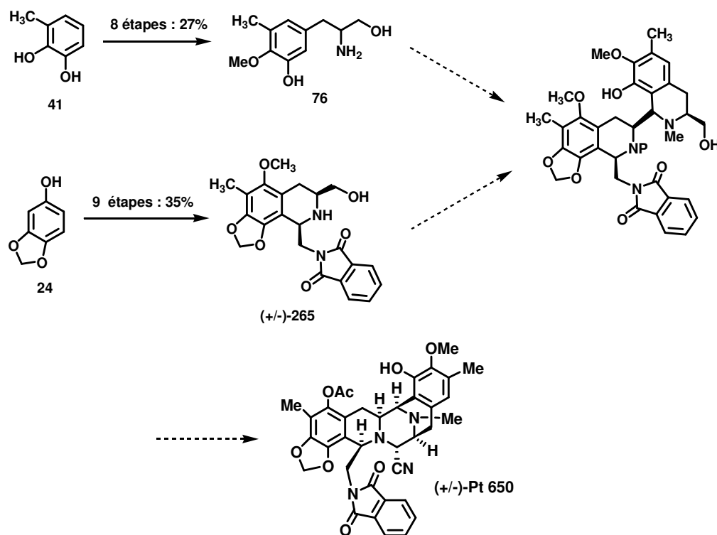
Schéma 66. Voie de synthèse vers ( \pm )-phthalascidine 650.
