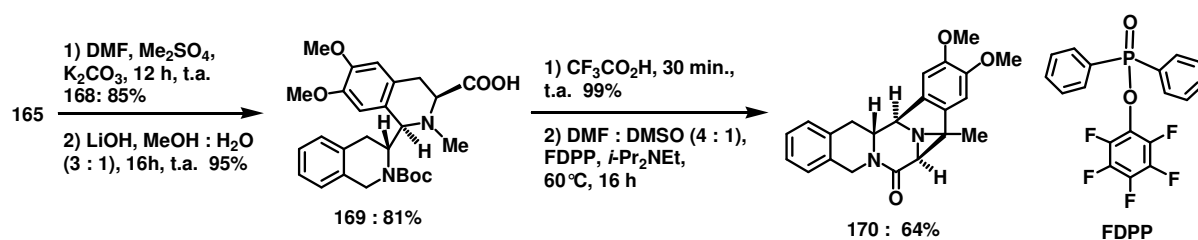
Schéma 34. Synthèse du lactame 170.
