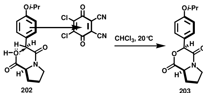
Schéma 46. Cyclisation intramoléculaire par oxydation benzylique asymétrique. 120a
