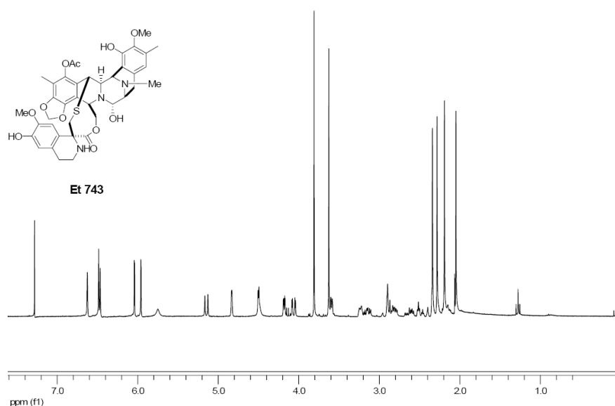
Figure 6. Spectre RMN du proton ^1\text{H} de l'ecteinascidine 743 (1). 5,23
