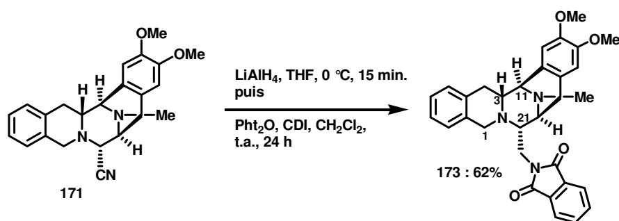
Schéma 36. Réduction de la fonction nitrile et fonctionnalisation de 171 .
