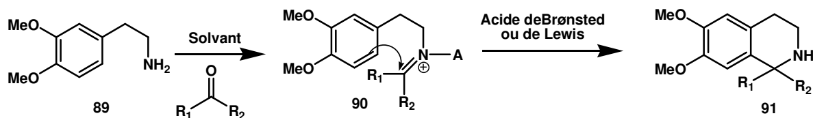
Schéma 13. Cyclisation par activation acide de l'intermédiaire imine.
