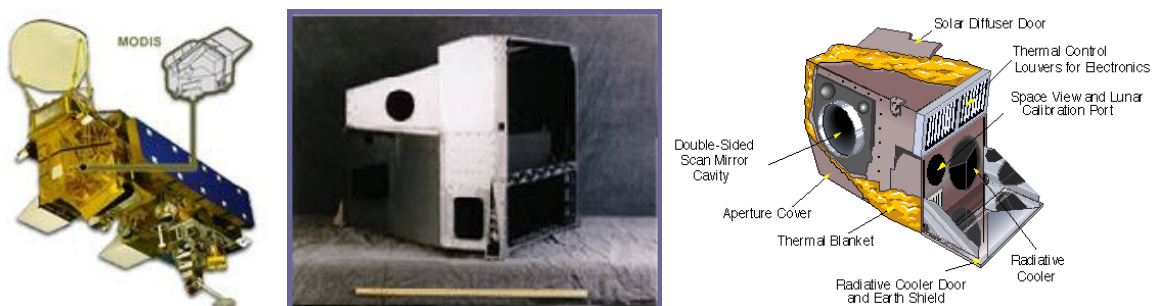
Figure 1.15 – A gauche, emplacement du capteur MODIS sur le satellite Aqua. Au milieu, photographie du capteur MODIS. A droite, schéma explicatif. [ http://modis.gsfc.nasa.org ]
