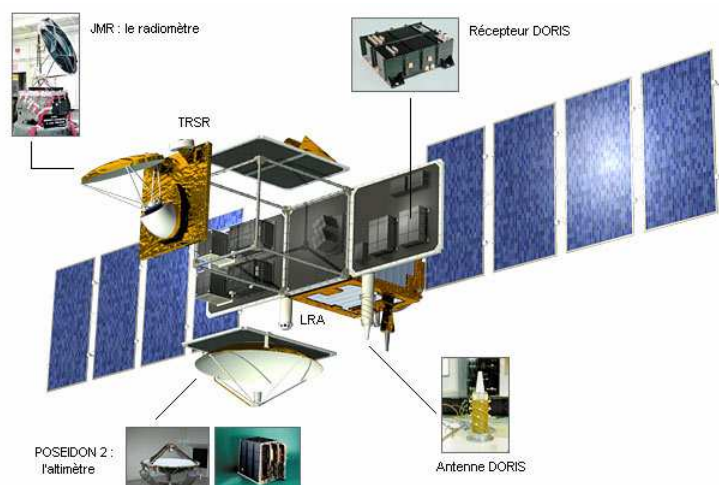
Figure A.8 – Positionnement des instruments à bords de Jason-1.
