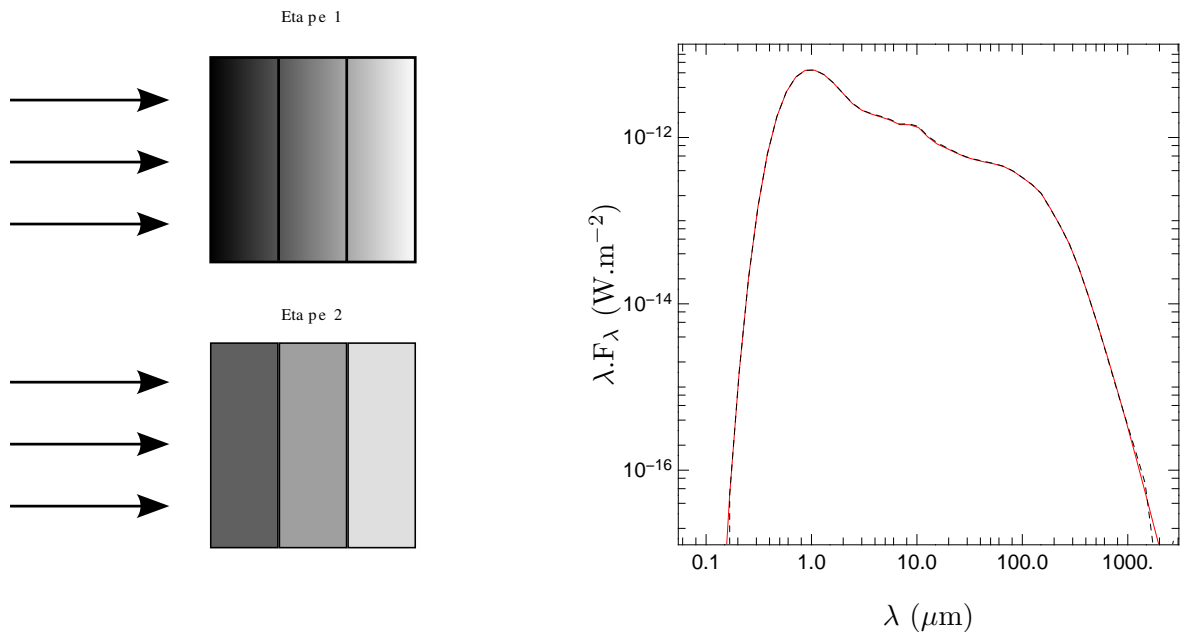
Figure 2.15 – Influence de la résolution de la grille spatiale au niveau du bord interne sur les distributions spectrales d'énergie simulées. Le panneau supérieur présente schématiquement le problème lié à une résolution insuffisante. Les carrés représentent une cellule au niveau du bord interne, la carte de couleur symbolisant la densité d'énergie thermique émise. Le rayonnement stellaire vient de la gauche et est représenté par les flèches. Lors de la première étape, la densité d'émission est par construction égale à la densité d'absorption et présente un fort gradient du bord interne vers le centre du disque. Dans la seconde étape, l'émission est supposée uniforme dans la cellule. Si la résolution est insuffisante, la différence entre les répartitions spatiales de l'émission thermique dans les deux étapes devient non négligeable et induit des erreurs au niveau de la distribution spectrale d'énergie. La courbe rouge représente le résultat produit par la seconde étape. Il est dans ce cas sensiblement différent de celui produit par la première étape (courbe noire en tirets). Le panneau inférieur présente le même calcul mais une augmentation de la résolution au bord interne. Les densités d'émission sont cette fois-ci beaucoup plus proches et les résultats des deux étapes sont en parfait accord.
