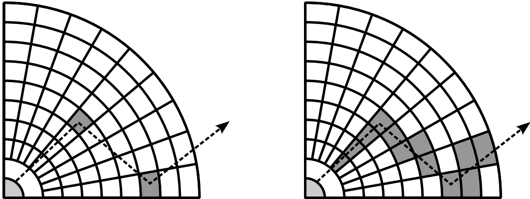
Figure 2.14 – Information créée par un photon lors de sa propagation. Dans la méthode Monte Carlo classique (figure de gauche), l'information n'est créée que dans les cellules où le photon interagit avec la matière. L'utilisation du concept d'intensité spécifique moyenne permet de produire de l'information dans toutes les cellules traversées par le photon (figure de droite), autorisant une diminution du nombre de photons nécessaires pour atteindre un certain degré de convergence, notamment dans les régions optiquement minces.
