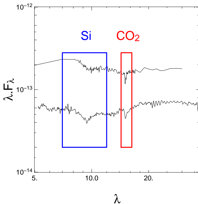
Figure 3.10 – Raies de silicates et de \text{CO}_2 en absorption observées dans le spectre de IRAS 04158+2805 (en bas). Le spectre observé n'a pas été calibré en absolu. Au-dessus, est décalé arbitrairement le spectre synthétique calculé en ajoutant des grains de \text{CO}_2 dans les zones du disque où la température est inférieure à 50 K.
