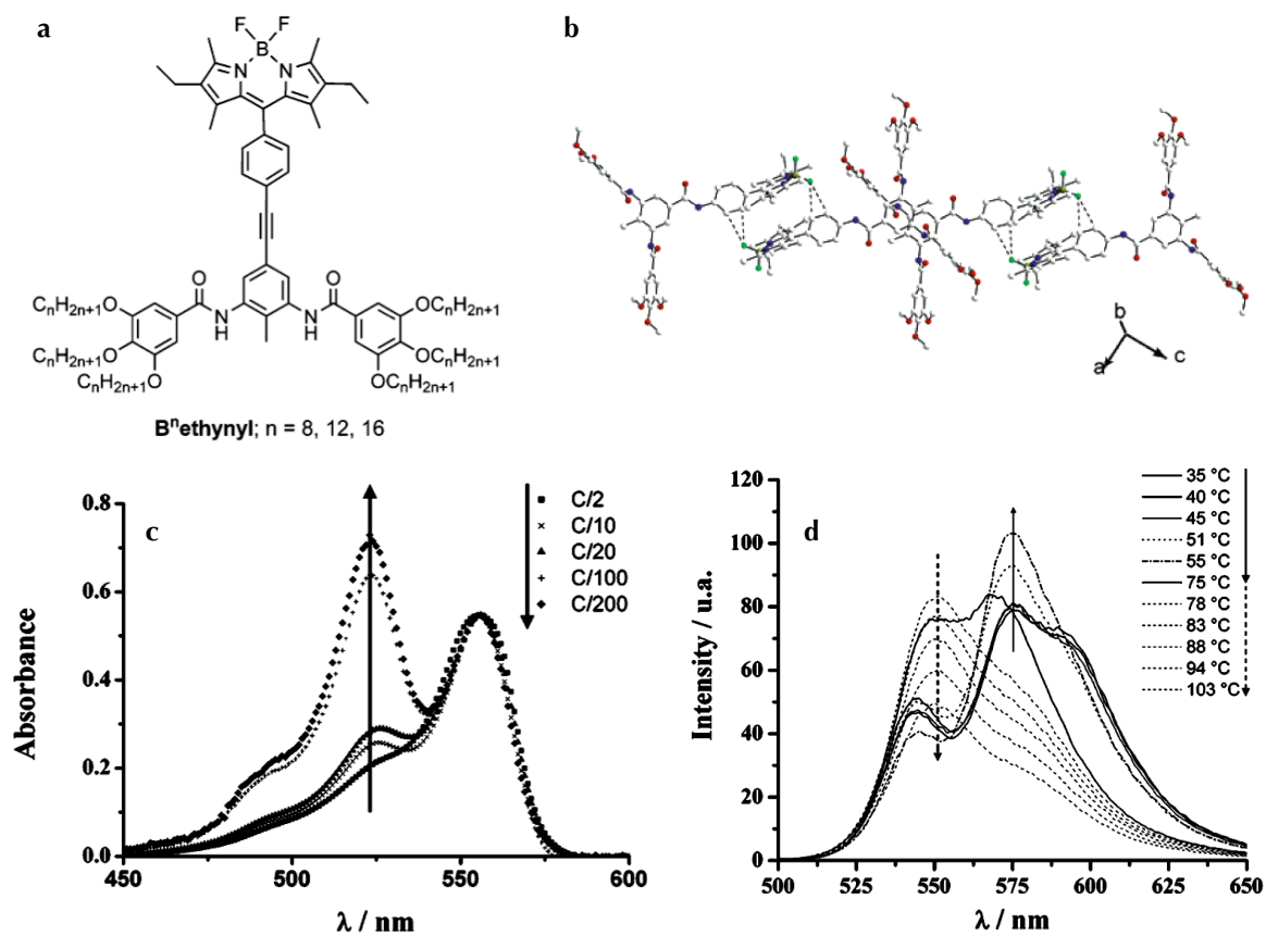
FIG. 3.17 – a) Structure des molécules B^n amide, b) Empilement des molécules, c) Spectres d'absorption du B^{16} amide dans le nonane à différentes concentrations, d) Spectres de fluorescence du B^{16} amide dans le nonane en fonction de la température, il y a formation d'un organogel. D'après [118]
