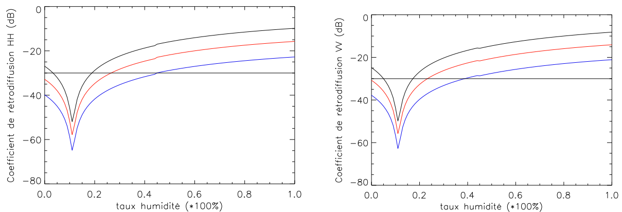
FIG. 6.32 – Variation des coefficients de rétrodiffusion \sigma_{S2hh}^2 (à gauche) et \sigma_{S2vv}^2 (à droite) en fonction de la teneur en eau du substratum basaltique pour une région de Mars présentant un contexte géologique défavorable (à forte concentration de roches, f = 0.08 ). Les simulations ont été réalisées pour un angle d'incidence \theta_i = 40^\circ et pour trois profondeurs de la couche de basalte : 1 m (en noir), 2 m (en rouge) et 3 m (en bleu) [Ph Paillou and Y. Lasne et al., 2005].
