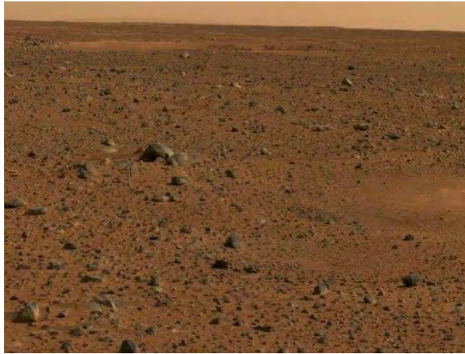
FIG. 6.22 – Image du site d’atterrissage du rover Spirit , dans la région du cratère de Gusev , révélant une distribution superficielle des roches similaire au cas de Chryse Planitia . Cette distribution correspond à un paramètre k = 0.05 pour le modèle de l’équation 6.6.
