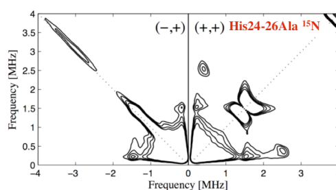
Figure 113 : Spectre HYSORE du double mutant His24-26Ala ^{15}\text{N} ( T = 15 \text{ K} , P = 1 \text{ mW} , enregistré dans la zone g_{\perp} ).
