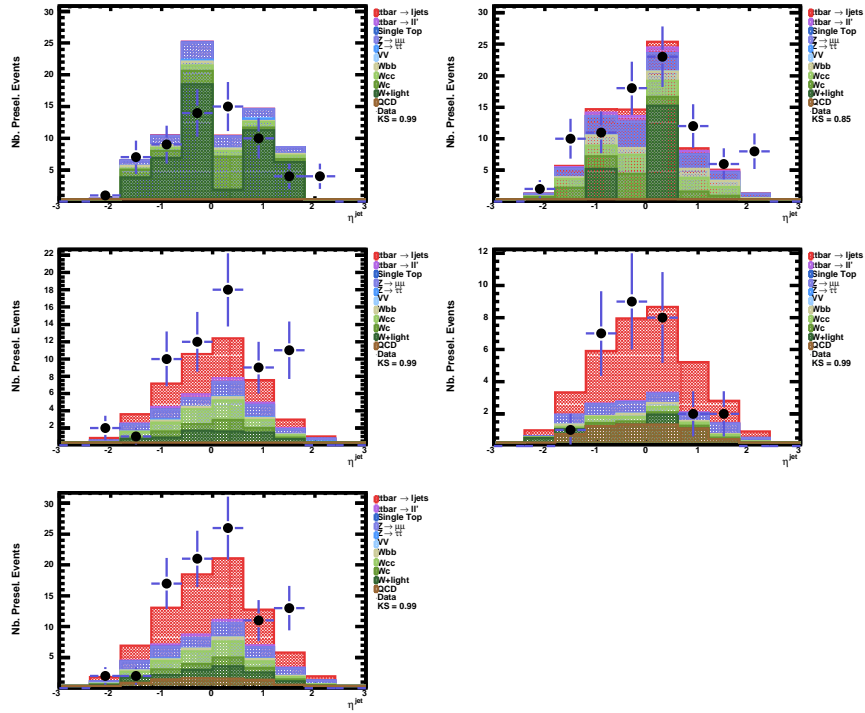
FIG. D.2.15 – Canal “muon+jets” : Pseudo-rapidité des jets.
