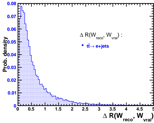
FIG. 7.2.7 – Distance \Delta R entre le boson W leptonique reconstruit et g n r .
