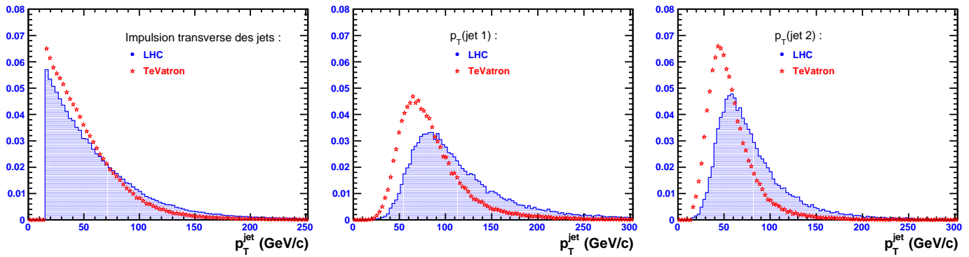
FIG. 1.3.14 – Impulsion transverse des jets dans les dans les événements t\bar{t} au TeVatron et au LHC pour : tous les jets reconstruits ( E_T^{\text{jet}} > 15 GeV et |\eta^{\text{jet}}| < 5 ) (à gauche), le jet de plus grande impulsion transverse (au centre), et le second jet de plus grande impulsion transverse (à droite).
