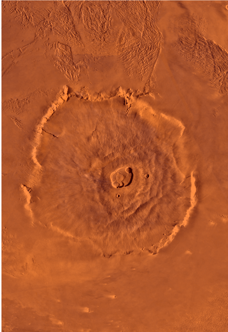
FIG. 6.14 – Image Viking d'Olympus Mons (Mosaïque MDIM 45N225). Les volcans boucliers majeurs de la région de Tharsis et d'Elysium se sont construits sur plusieurs milliards d'années suite à de nombreux cycles effusifs comme en témoignent leurs calderas complexes. La largeur de l'image couvre 780 km.
