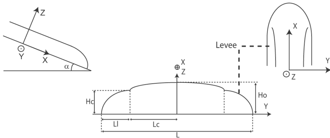
FIG. 5.15 – Schéma de la coulée au début de l'écoulement avec le repère. L'écoulement se fait dans le plan (x, y) , 'x' étant orienté suivant la ligne de plus grande pente. L =Largeur totale de la coulée, L_l =Largeur des levées, 2L_c =Largeur de l'écoulement, H_c =Hauteur critique, H_o =épaisseur de la lave au centre de la coulée.
