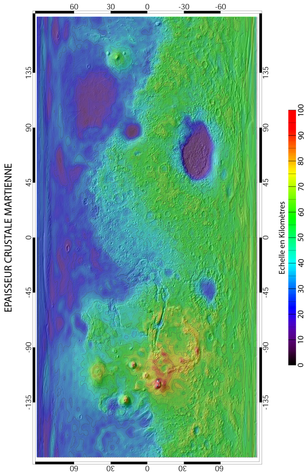
FIG. 5.5 – Epaisseur de la croûte Martienne dérivée des données topographiques et gravimétriques [Wieczorek et Zuber, 2004]. Noter que le dôme de Tharsis présente une épaisseur de 80 km environ, alors que le manteau Martien se trouve à moins de 10 km du plancher du bassin d'impact de Hellas. L'épaisseur moyenne de croûte dans les Highlands du sud est de 60 km alors que dans les Lowlands du nord, l'épaisseur crustale moyenne est de 20 km.
