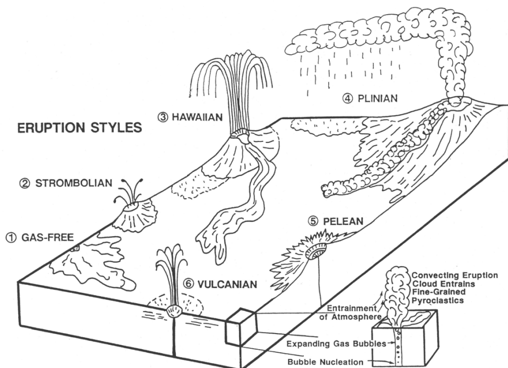
FIG. 5.12 – Variétés des styles d'éruptions sur Terre que l'on peut utiliser pour la description du volcanisme martien : (1) 'Gaz free' correspond à des coulées de laves effusives sans gaz, et donc sans phénomène explosif. (2) Le volcanisme Strombolien est un événement explosif et effusif au cours duquel le magma voit alternativement sa vitesse augmenter, autorisant de façon intermittente, la formation de grosses bulles de gaz. (3) le volcanisme Hawaïien est composé de larges pyroclastes et de coulées de laves rapidement séparées du gaz. (4) Les éruptions Pliniennes développent de petits pyroclastes qui forment des nuages d'ignimbrites en fonction de la densité du mélange (pyroclastique, gaz, gaz atmosphériques). (5) Les éruptions Peléennes ont des compositions de magmas allant de acide (riche en silice) à intermédiaire. Le gaz peut être piégé dans la lave refroidissant de façon désordonnée. (6) Le volcanisme Vulcanien résulte d'interactions de type eau-magma et glace-magma. Sur Mars, c'est ce dernier volcanisme qui est le plus susceptible de se produire en raison de la proportion de glace présente dans le sol martien. D'après Wilson et Head , [1994]
