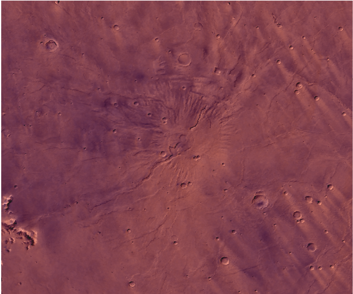
FIG. 6.12 – Image Viking de Tyrrhena Patera (Mosaique MDIM 45S135). Ces volcans plats d'apparences explosives sont typiques des highlands et d'un volcanisme ancien de Mars. Les reliefs sont très érodés, les calderas difficiles à définir et les flancs des édifices présentent des signes d'écoulements d'eau suggérant des possibles interactions phréato-magmatiques. La largeur de l'image couvre 660 km de surface martienne.
