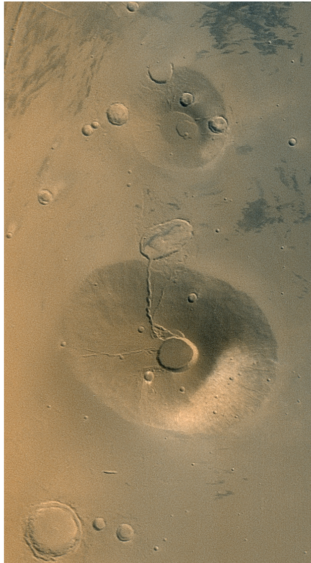
FIG. 6.10 – Image MOC grand angle (E14-1248-1249) de Ceraunius Tholus (100 km de diamètre à la base) et Uranus Tholus en haut. Ces petits édifices volcaniques de Tharsis sont les reliques d'un volcanisme Noachien.
