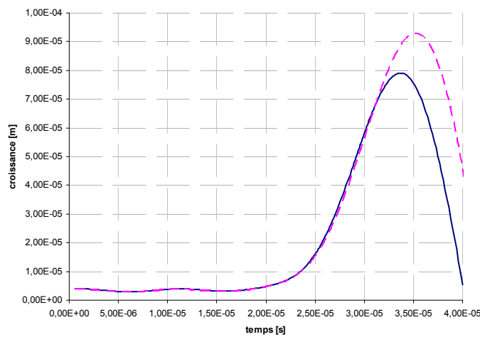
figure 2-32 : Croissance de l'instabilité en prenant en compte (Sp) ou non (S0) l'augmentation de la surface d'échange
