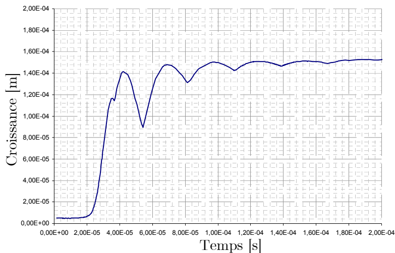
figure 2-14 : Croissance maximale des instabilités en \eta = \eta_0 |F|
