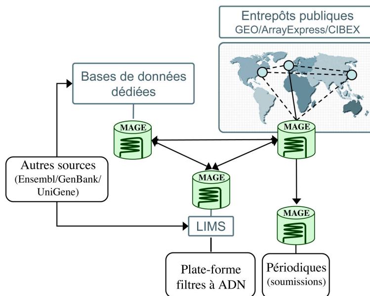
FIG. 2.15 – Agencement possible entre les différentes bases de données. L'ensemble des transactions entre les différentes sources de données de puces à ADN est effectuée idéalement par l'intermédiaire du MAGE. Ainsi, associés aux plate-formes de puces à ADN des laboratoires, les LIMS peuvent d'une part récupérer les informations soit auprès de sources diverses telles UniGene soit auprès de bases de données dédiées (idéalement grâce au MAGE), et d'autre part déposer les résultats d'expériences dans les conservatoires publics. Ces derniers permettent alors aux auteurs de soumettre leurs travaux aux périodiques scientifiques.
