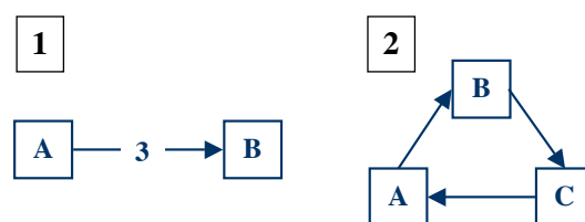
FIG. 3.3 – Représentation graphique . Chaque carré représente un paramètre à étudier. Chaque flèche représente une comparaison. (1) La comparaison directe de A et B est effectuée par trois répliques techniques. (2) A et B sont comparables suivants deux chemins : l'un direct de longueur 1 ( \log(\frac{A}{B}) ) et l'autre indirect de longueur 2 mais en conséquence moins précis ( \log(\frac{A}{C}) - \log(\frac{B}{C}) ).
