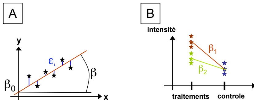
FIG. 3.5 – Regression lineaire . A. Régression linéaire simple. En bleu sont représentées les distances \epsilon_i entre les valeurs y observées et les valeurs \hat{y} estimées par la méthode des moindres carrés. La droite en brun est la représentation de l'équation \hat{y} = \beta_0 + \beta x , dont \beta est le coefficient directeur et \beta_0 est le terme d'intersection. B. Régression linéaire multiple. Les points en vert et brun représentent les valeurs expérimentales de deux traitements à comparer aux valeurs expérimentales d'un contrôle. Pour chaque traitement le coefficient directeur de la droite de régression linéaire peut-être estimé par la méthode des moindres carrés.
