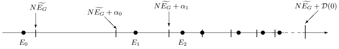
FIG. 4.2 – Relation entre les spectres de la matrice M et de l'opérateur H_{\text{exc}} . \widetilde{E}_G , \mathcal{D}(0) et \gamma_n dépendent de \lambda .
