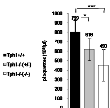
Figure 56: Nombre total de plaquettes sanguines chez les souris Tph1 -/+ , Tph1 -/- vs. Tph1 +/+ (commerce). Les mesures ont été effectuées sur des animaux âgés de 20 semaines. n=6 souris dans chaque groupe. Les résultats sont exprimés en moyenne ± déviation standard. *p<0.05, ***p<0.001.
