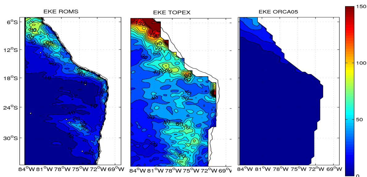
Figure 2.5 : Energie cinétique turbulente (EKE) moyenne évaluée à partir de ROMS (gauche), TOPEX (milieu), ORCA05 (droite). L'unité est le \text{cm}^2/\text{s}^2 .
