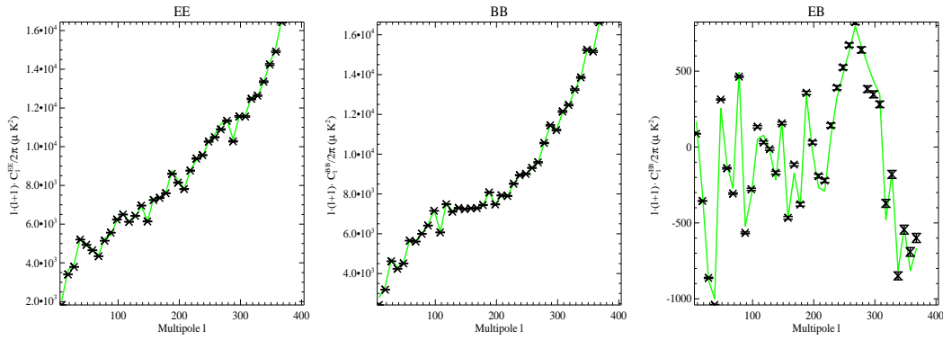
FIG. 9.21 – Reconstruction CMB-fixé en polarisation de l’émission synchrotron, à partir de simulations [planck d] de cartes Q et U . Les spectres C_\ell^{EE} , C_\ell^{BB} and C_\ell^{EB} sont présentés en \mu\text{K}_{\text{CMB}}^2 à 30 GHz (croix). Le modèle d’entrée est superposé en vert. Les barres d’erreur correspondent à la dispersion sur 100 simulations.
