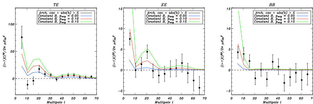
FIG. 7.6 – Spectres de puissance angulaire C_l^{TE} (gauche), C_l^{EE} (centre) et C_l^{BB} (droite), en \mu K_{RJ}^2 , calculés à partir des données à 353 GHz de l'expérience ARCHEOPS (points noirs), pour une coupure |b| \geq 5 . Nous leur comparons les spectres calculés à l'aide de notre modèle d'émission galactique simplifié (voir texte ci-dessus), pour différents degrés de polarisation de la poussière, 5 (bleu), 10 (rouge) et 15% (vert).
