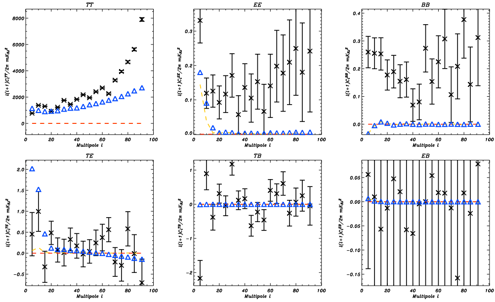
FIG. C.16 – Spectres de puissance angulaire C_{\ell}^{TT} , C_{\ell}^{EE} , C_{\ell}^{BB} , C_{\ell}^{TE} , C_{\ell}^{TB} et C_{\ell}^{EB} (de gauche à droite et de haut en bas), en \mu K_{\text{CMB}}^2 calculés par la méthode décrite en 10.6.2 à partir des cartes I , Q et U mesurées par WMAP à 61 GHz [Page et al. 2006] et auxquels nous avons soustrait le bruit instrumental à l'aide de simulations (croix noires). Les barres d'erreurs sont également estimées à partir des simulations de bruit. Nous leur comparons les spectres de puissance angulaire de notre "modèle raffiné" extrapolé à 61 GHz, pour le synchrotron (ligne brisée orange) et pour la poussière (ligne brisée rouge). Nous présentons également la somme de ces deux composantes à laquelle nous avons ajouté une contribution de CMB et de rayonnement de freinage (triangles bleus). Ces spectres sont calculés pour une coupure galactique |b| > 10 .
