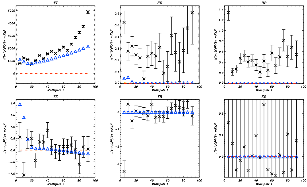
FIG. C.17 – Spectres de puissance angulaire C_{\ell}^{TT} , C_{\ell}^{EE} , C_{\ell}^{BB} , C_{\ell}^{TE} , C_{\ell}^{TB} et C_{\ell}^{EB} (de gauche à droite et de haut en bas), en \mu K_{\text{CMB}}^2 calculés par la méthode décrite en 10.6.2 à partir des cartes I , Q et U mesurées par WMAP à 94 GHz [Page et al. 2006] et auxquels nous avons soustrait le bruit instrumental à l'aide de simulations (croix noires). Les barres d'erreurs sont également estimées à partir des simulations de bruit. Nous leur comparons les spectres de puissance angulaire de notre "modèle raffiné" extrapolé à 94 GHz, pour le synchrotron (ligne brisée orange) et pour la poussière (ligne brisée rouge). Nous présentons également la somme de ces deux composantes à laquelle nous avons ajouté une contribution de CMB et de rayonnement de freinage (triangles bleus). Ces spectres sont calculés pour une coupure galactique |b| > 10 .
