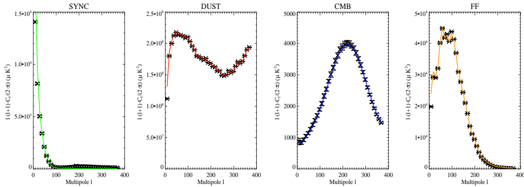
FIG. 9.18 – Reconstruction en température seule des spectres C_\ell^{TT} (croix) en \mu\text{K}_{\text{CMB}}^2 dans le cas d'une séparation A-fixée des simulations [planck d] pour les quatre composantes physiques. De gauche à droite : synchrotron (à 30 GHz), poussière- réaliste (à 353 GHz), CMB (à 100 GHz) et rayonnement de freinage (à 30 GHz). Les modèles d'entrée y sont superposés en lignes pleines, pour chacune des composantes. Les barres d'erreur correspondent à la dispersion sur 100 simulations.
