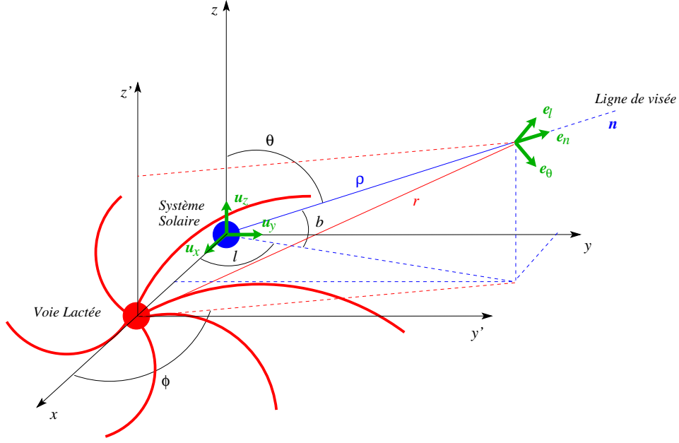
FIG. 10.1 – Définition des repères galactocentrique et de la ligne de visée que nous utiliserons au cours de ces travaux.
