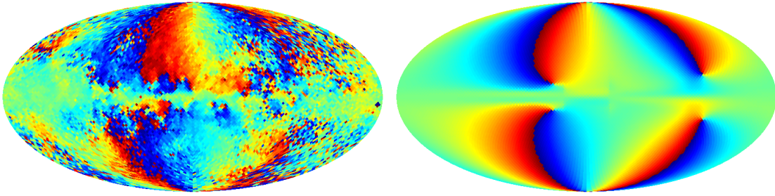
FIG. 10.4 – Gauche : Carte du ciel de l'angle de polarisation \gamma^{\text{WMAP}} calculé à partir des cartes WMAP à 23 GHz [Page et al. 2006], à partir de l'équation (10.14). Droite : Carte du ciel de l'angle de polarisation \gamma^{\text{modèle}} calculé à partir du “modèle raffiné” pour les paramètres définis en (10.16). Pour ces deux cartes, l'angle de polarisation est compris entre -\pi/2 (bleu) et \pi/2 (rouge). Nous pouvons observer une très bonne adéquation entre le modèle et les données.
