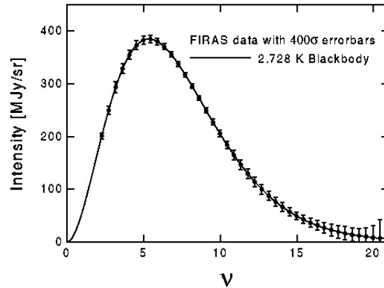
FIG. 2.1 – Spectre en fréquence de la puissance rayonnée par le CMB. Le modèle de corps noir est représenté en ligne pleine. Notons que les barres d'erreur ont été multipliées par 400 pour être visibles.
