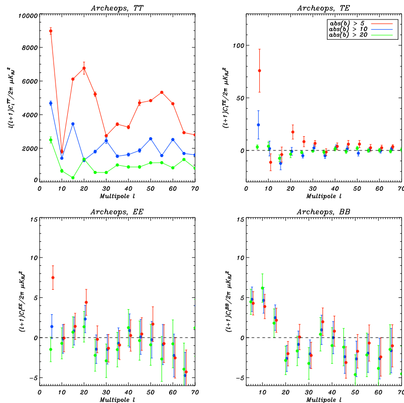
FIG. 7.3 – Spectres de puissance angulaire C_\ell^{TT} , C_\ell^{TE} , C_\ell^{EE} et C_\ell^{BB} en \mu\text{K}_{RJ}^2 calculés à partir des données à 353 GHz de l'expérience ARCHEOPS, pour trois coupures galactiques différentes, |b| = 5 (rouge), 10 (bleu) et 20 degrés (vert).
