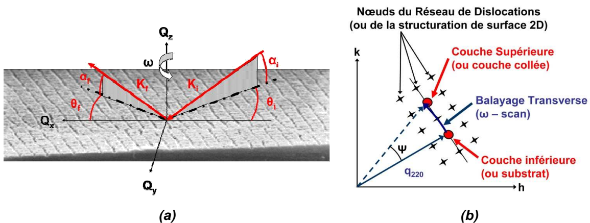
Figure III-43 : (a) Schéma des angles et vecteurs utilisés en diffraction des rayons X en incidence rasante. (b) Espace réciproque autour de la raie (220) dans le référentiel moyen. Les croix noires représentent les nœuds du réseau réciproque du réseau de dislocations enterrées (ou de la structuration de surface 2D). Les deux ronds rouges symbolisent les pics de Bragg de la couche collée (couche supérieure) et du substrat (couche inférieure). L'arc de cercle est le trajet du transfert de moment lors d'un balayage angulaire suivant \omega (appelé \omega -scan).
