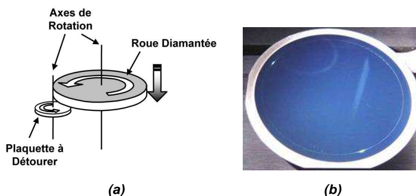
Figure II-10 : (a) Schéma de principe du détournage. La roue diamantée et la plaque à détourer tournent en sens contraire. La roue descend graduellement abrasant la périphérie de la plaque et s'arrête à une côte donnée avec une précision de 1 \mu\text{m} . (b) Photo d'un Négatif détourné avec l'échelle graduée en périphérie de la plaque.
