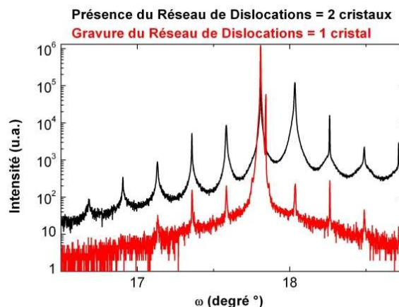
Figure III-45 : Balayages angulaires \omega -scan autour de la raie (220) sur un même échantillon avec deux niveaux de gravure différents : pour la courbe noire, la gravure s'est arrêtée avant d'atteindre le réseau de dislocations (environ +5 nm) et pour la courbe rouge, la gravure s'est arrêtée au-delà du réseau de dislocations (environ -5 nm). \alpha_i = \alpha_f = 0,24^\circ et E = 10 keV.
