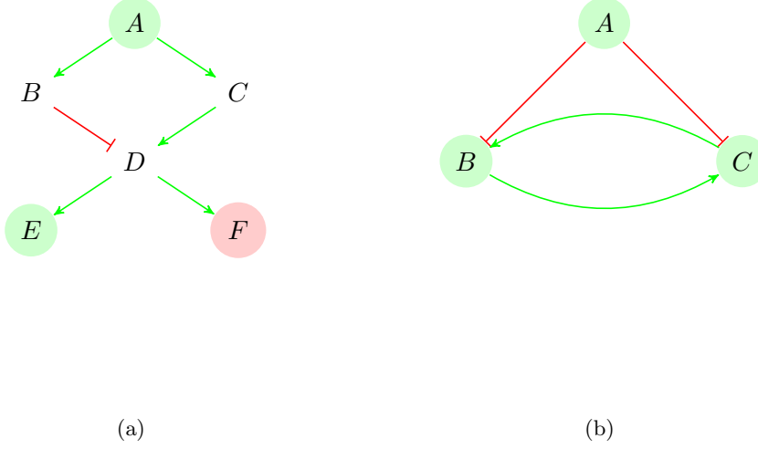
FIG. 7.2 – Contre-exemples pour la preuve du théorème 12. (a) Cas \mathcal{P} -consistant mais pas \mathcal{N} -consistant. (b) Cas \mathcal{N} -consistant mais pas \mathcal{P} -consistant. Les deux graphes ont une seule entrée : A .
