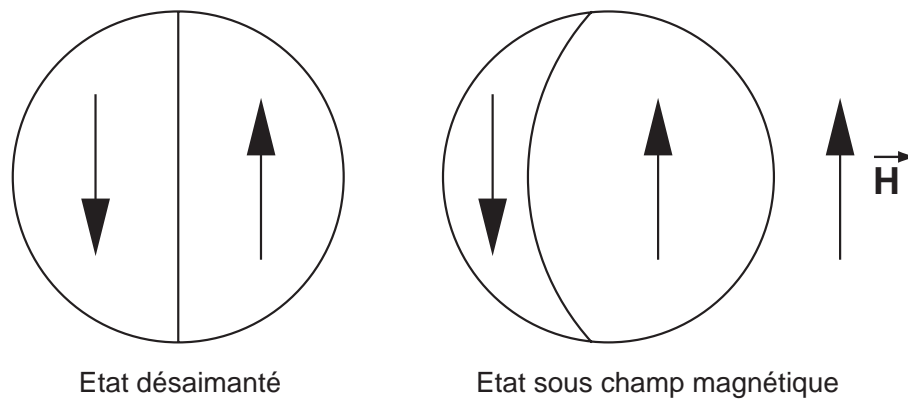
FIG. A.1: Modèle de Globus à l'échelle du grain
