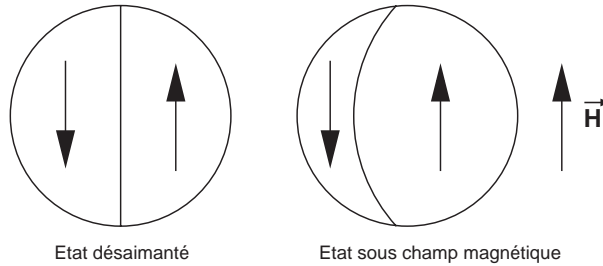
FIG. 4.3: Modèle de Globus à l'échelle du grain
