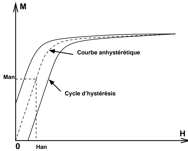
(a) Point mesuré de la courbe anhystérétique
