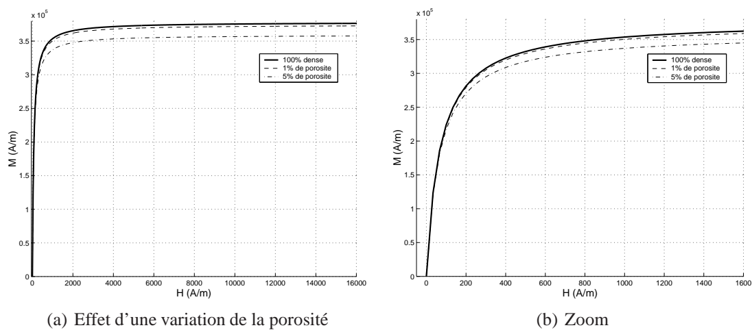
FIG. A.8: Comportement magnétique en fonction de la porosité
