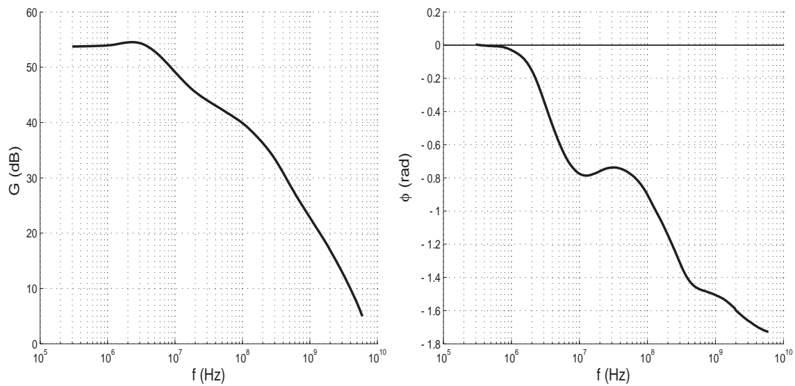
FIG. 2.26: Diagrammes de Bode en gain ( G ) et en phase ( \phi ) de la perméabilité du ferrite Ni-Zn
