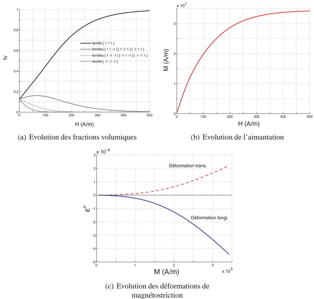
FIG. 3.12: Comportement du monocristal sans contrainte appliquée avec \vec{H} // [111]
