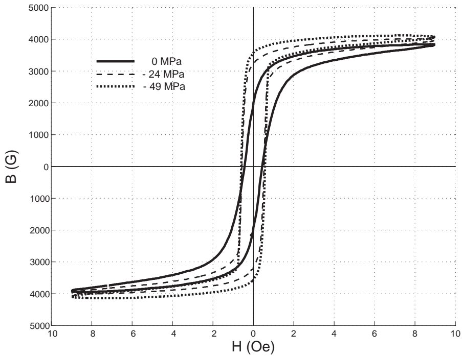
FIG. 2.22: Comportement magnétique du tore en compression radiale
