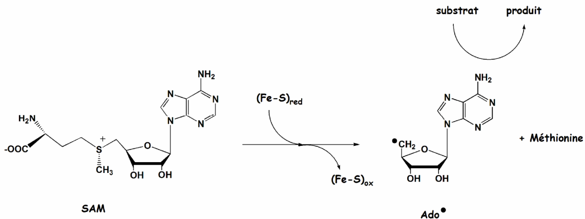
Figure 3 : Equation bilan de la réductolyse de la SAM
