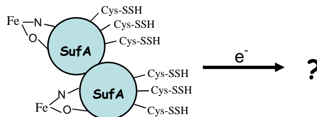
Figure I-45 : représentation schématisée de la réaction étudiée ; -SSH représente les persulfures sur les cystéines de SufA, le fer étant localisé ailleurs dans la protéine, coordonné par des atomes d'azote et d'oxygène.
