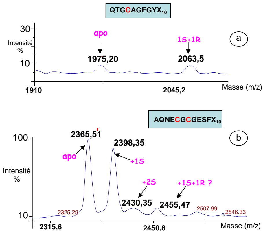
Figure I-41 : spectres MALDI de SufA-SSH après traitement avec 25 excès molaires d'iodoacétamide et digestion par l'endoprotéinase Lys-C. Seuls les spectres des peptides [47-65] (a) et [110-130] (b) sont représentés.
