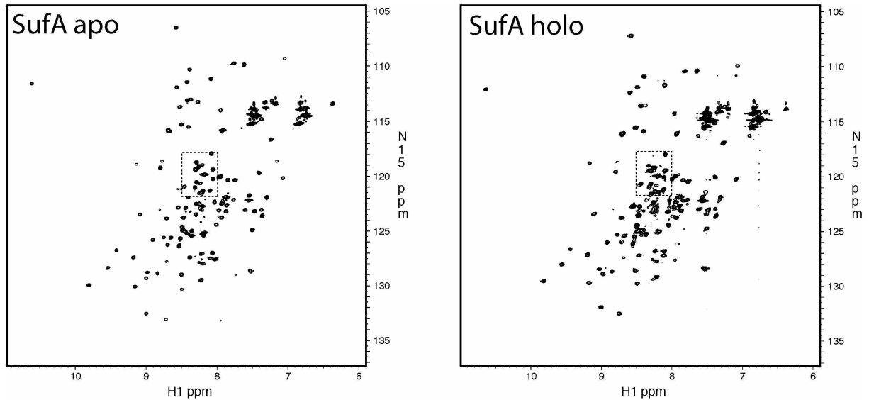
Figure III-4 : comparaison des spectres HSQC des protéines SufA apo et holo, enregistrés à 600 MHz, à 25°C. Le rectangle en pointillé correspond à la région contenant les tâches de résonance des cystéines conservées. Un zoom de cette région est représenté dans la figure suivante (III-5). SufA apparaît ici comme un monomère car les tâches de résonance des deux sous-unités du dimère sont superposables.
