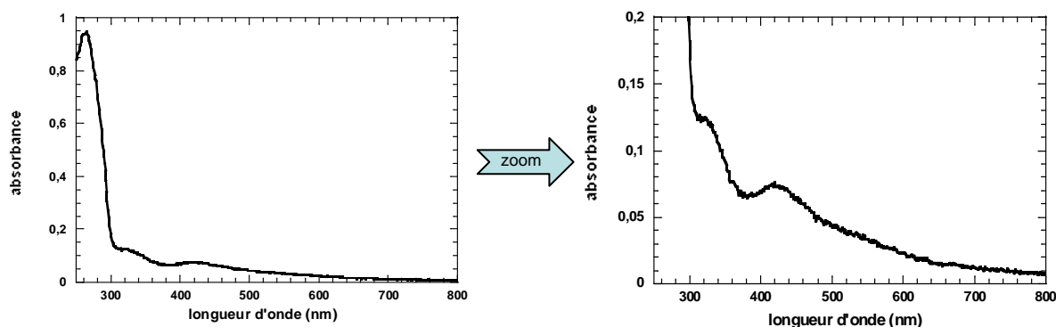
Figure II-7 : spectre UV-visible de SufA (70 μM) obtenue après purification en anaérobiose à partir du plasmide pGSO 164 SufD_H128A codant pour l'ensemble de l'opéron suf , enregistré dans une cuve de 1 cm de trajet optique.
