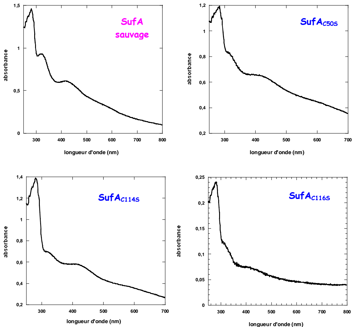
Figure III-1 : spectres UV-visible des protéines SufA C50S (110 μM), SufA C114S (120 μM) et SufA C116S (17 μM) obtenues après reconstitution chimique puis dessalage (conditions utilisées ici : 4 excès molaires de fer et de soufre inorganiques, temps d’incubation 3 heures). Le spectre obtenu pour la protéine SufA sauvage (125 μM) dans les mêmes conditions est représenté pour comparaison.
