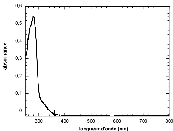
Figure I-9 : Spectre d'absorption UV-visible de la protéine SufA sauvage (35 \mu M) enregistré avec une cuve de 1 cm de trajet optique, dans le tampon Tris-HCl 50 mM pH 7,5, NaCl 100 mM, DTT 5 mM.
