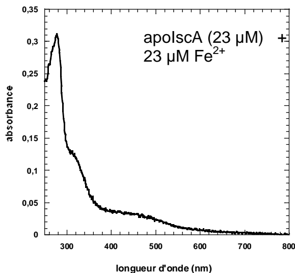
Figure I-33 : spectre UV-visible de IscA (23 µM) après incubation avec 1 excès molaire de Fe(II) et dessalage en conditions anaérobies
