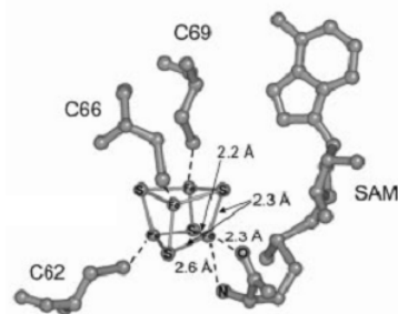
Figure 2 : Structure obtenue aux rayons X (2,07 Å) du site actif ([Fe-S] + SAM) de Hem N, une protéine de la famille radical-SAM (Layer et al. , 2005)
