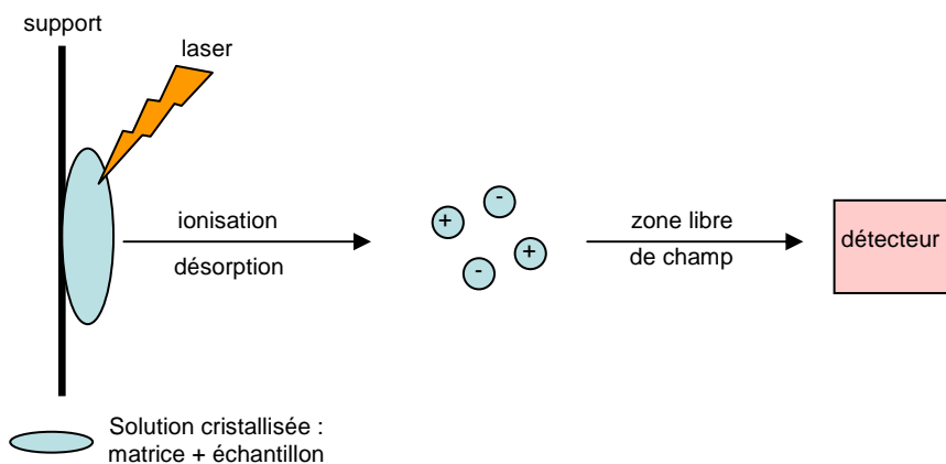
Figure 22 : principe de la spectrométrie MALDI
