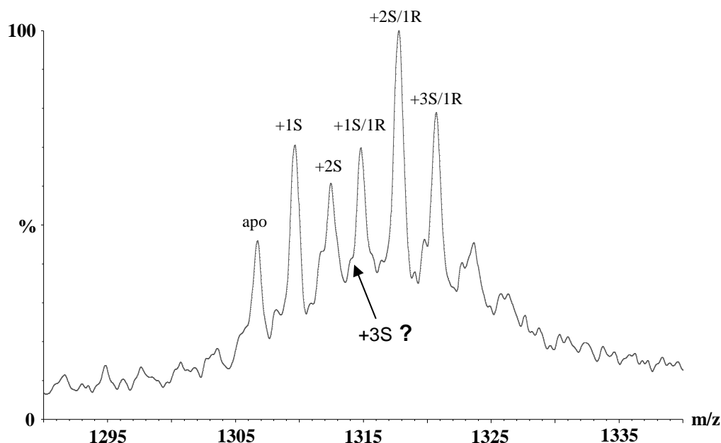
Figure I-39 : spectre de masse de SufA (500 nM) après transfert de soufre depuis le complexe SufSE et traitement avec 25 excès molaires d'iodoacétamide à température ambiante puis dessalage (S= atome de soufre ; R = groupement acétamide). Seul l'état de charge z=11 est représenté.
