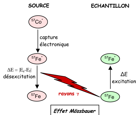
Figure 18 : Principe de l'effet Mössbauer
