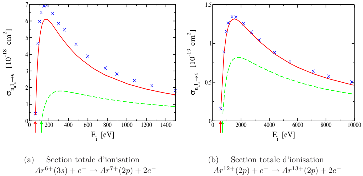
FIG. 4.11 – Sections efficaces totales d'ionisation collisionnelles écrantées (—), non écrantées (- -) et partiellement écrantées (×) (voir texte) pour deux ions argon. Les sections écrantées sont calculées avec l'expression (4.79) pour une densité électronique de 10^{23} \text{ cm}^{-3} et une température de 30 eV. Les flèches indiquent l'énergie seuil de la transition.
