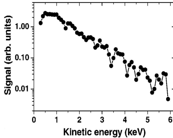
FIG. 1.7 – Distribution en énergie des électrons émis lors de l'interaction entre une impulsion laser (400 fs; 10^{16} W.cm -2 ) et des agrégats de xénon ( 2,4 \times 10^6 atomes/agrégat) [Springate et al. 03].
