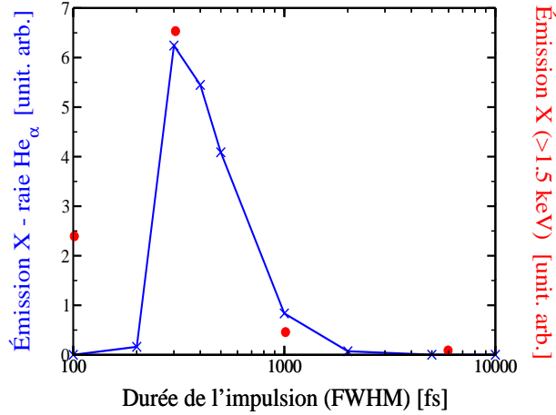
FIG. 5.9 – (×—×) Variation de l'émission X pour la raie He_\alpha (3,14 keV) en fonction de la durée d'impulsion. Ces résultats ont été obtenus pour une énergie par impulsion de 50 mJ et une longueur d'onde de 800 nm. Le rayon de l'impulsion en 1/e de l'intensité est de 10\ \mu\text{m} , ce qui donne un éclairement crête de 1,3 \times 10^{17}\ \text{W}\cdot\text{cm}^{-2} pour une durée d'impulsion à mi-hauteur de 100 fs. (•) Données expérimentales obtenues par E. Parra et coll. pour l'émission X supérieure à 1,5 keV [Parra et al. 00].
