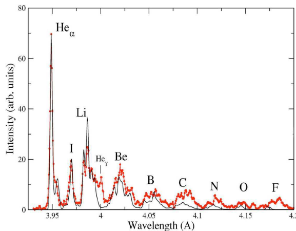
FIG. 1.10 – Spectre expérimental (●—●) et théorique (—) obtenus pour des agrégats d'argon de 1 \mu\text{m} irradiés par une impulsion laser ( \tau_{FWHM} = 30 \text{ fs} ; I_0 = 10^{19} \text{ W.cm}^{-2} ). Le spectre théorique a été obtenu avec N_a = 3,162 \times 10^{20} \text{ cm}^{-3} et \delta\tau = 5,7 \text{ ps} (voir texte pour explications) [Sherrill M. et al. 06].
