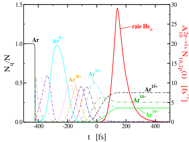
FIG. 5.18 – (—) Dynamique théorique de la raie \text{He}_\alpha pour l'interaction d'un agrégat d'argon ( R=275 Å) irradié par une impulsion laser ( \tau_{FWHM}=300 fs; I_0=3,1\times 10^{16} W.cm ^{-2} ; E=3,5 mJ). Les évolutions temporelles des populations de chaque état de charge (normalisées au nombre d'atomes dans l'agrégat) sont également représentées. Le temps t=0 fs correspond à l'instant où le champ laser est maximal.
