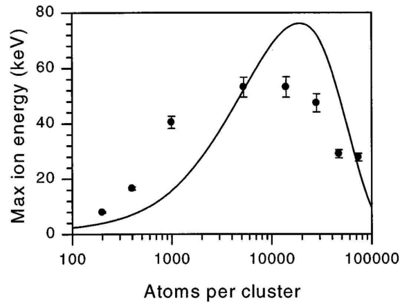
FIG. 1.8 – Énergie ionique maximale obtenue expérimentalement (●) et théoriquement (—) en fonction de la taille des agrégats de xénon irradiés par une impulsion laser de 230 fs et 3 \times 10^{15} \text{ W.cm}^{-2} [Springate et al. 00].
