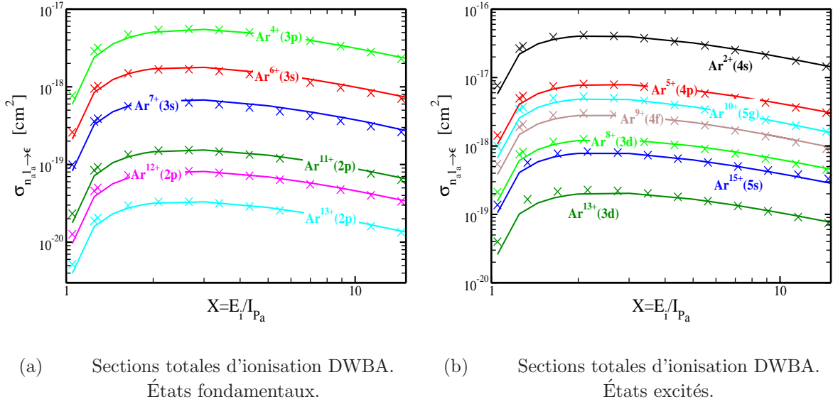
FIG. 3.5 – (—) Sections efficaces totales d'ionisation collisionnelles dans l'approximation des ondes distordues (éq. (3.129)) pour des ions Ar^{q+} (états fondamentaux ou excités). Les sections moyennées sur les sous-niveaux magnétiques sont représentées en fonction du rapport X de l'énergie de l'électron incident E_i au potentiel d'ionisation du niveau considéré I_{Pa} = |E_a| et comparées aux données de référence ( \times ) [IAEA].
