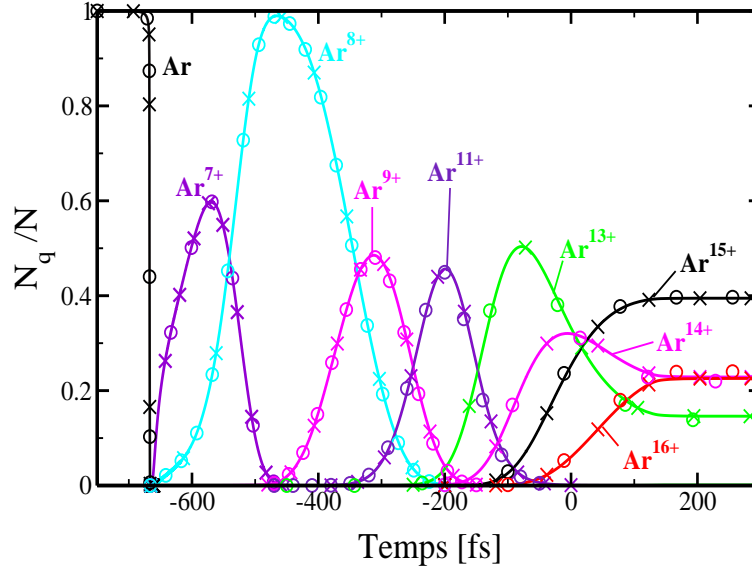
FIG. 5.3 – Évolution temporelle des populations totales N_q normalisées au nombre initial d'atomes dans l'agrégat pour certains états de charge Ar^{q+} . (—) Résultats obtenus en considérant l'évolution de couches d'états n . (x) Résultats obtenus en considérant l'évolution d'états excités nl . (o) Résultats obtenus en considérant jusqu'à 8 couches d'états excités (voir texte). Les conditions de l'interaction sont identiques à celles de la figure 5.1.
