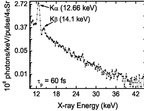
FIG. 1.4 – Spectre X obtenu en irradiant des agrégats de krypton ( R_0 \sim 18 nm) par une impulsion laser de 60 fs et un éclairement crête de 1,3 \times 10^{18} W.cm -2 [Issac et al. 04].
