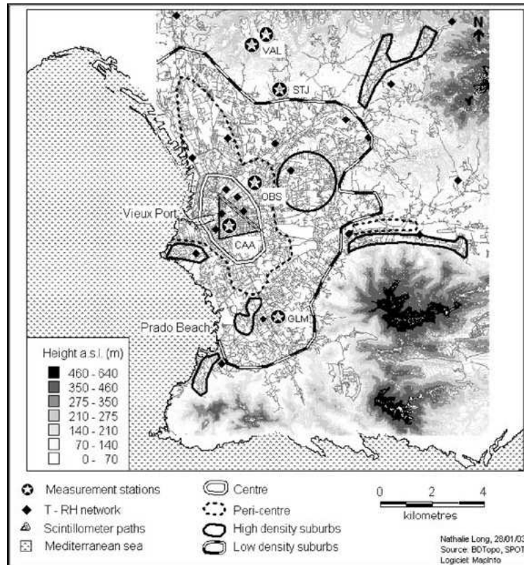
FIG. 2.1: Dispositif expérimental de la campagne CLU-ESCOMPTE sur un fond de carte de l'agglomération marseillaise ( Mestayer et al., 2005 ). Les étoiles indiquent les stations de bilan d'énergie; les losanges, le réseau urbain de mesures de température et d'humidité; et les lignes, le trajet optique du scintillomètre. Les limites des différentes zones urbaines sont indiquées d'après les travaux de Long (2003) .
