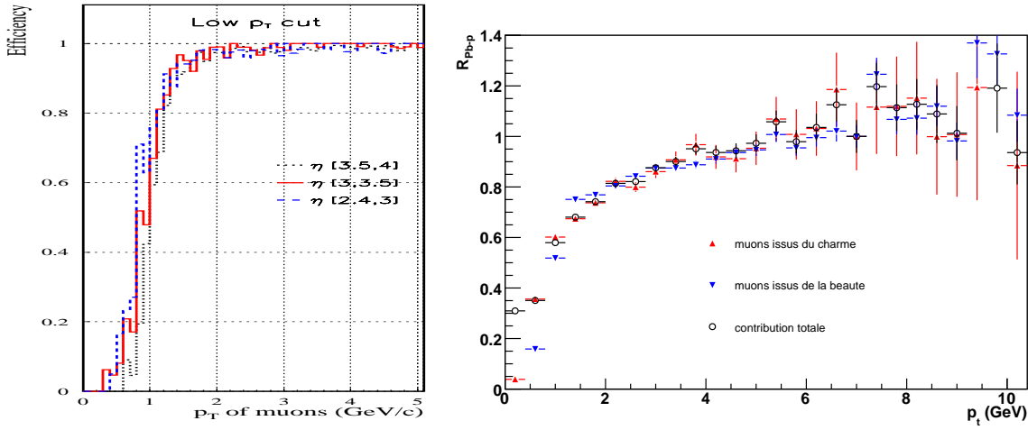
FIG. 7.23 – Efficacité du système de déclenchement en fonction de p_t (figure de gauche) et rapport des distributions des muons en tenant compte des coupures cinématiques et l’acceptance du spectromètre à muons (figure de droite).
