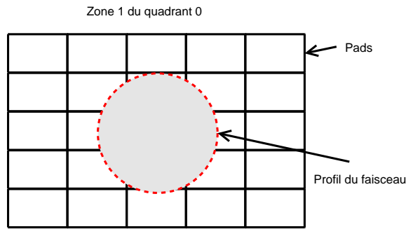
FIG. 5.6 – Profil du faisceau sur le plan non-bending du quadrant 0 de la station 1.
