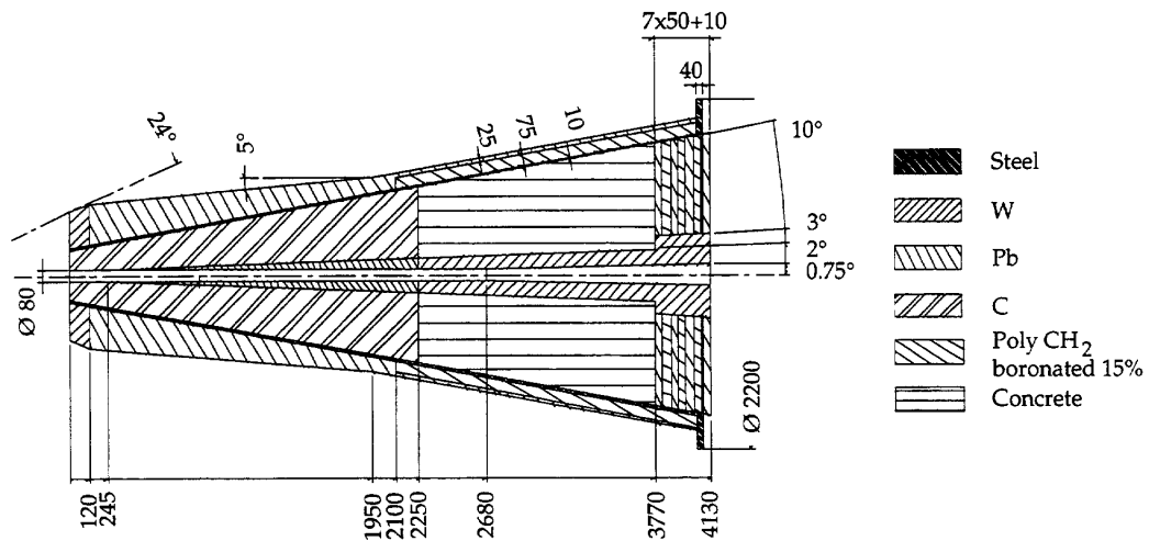
FIG. 3.13 – Vue en coupe de l'absorbeur frontale du spectromètre à muons du détecteur ALICE.
