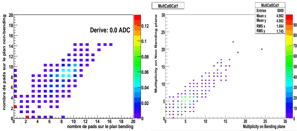
FIG. 6.6 – Multiplicité des pads des clusters sur chacun des plans de cathode obtenue en simulation (à gauche) et en conditions expérimentales (à droite). Ces résultats sont associés aux quadrants de la station 1.
