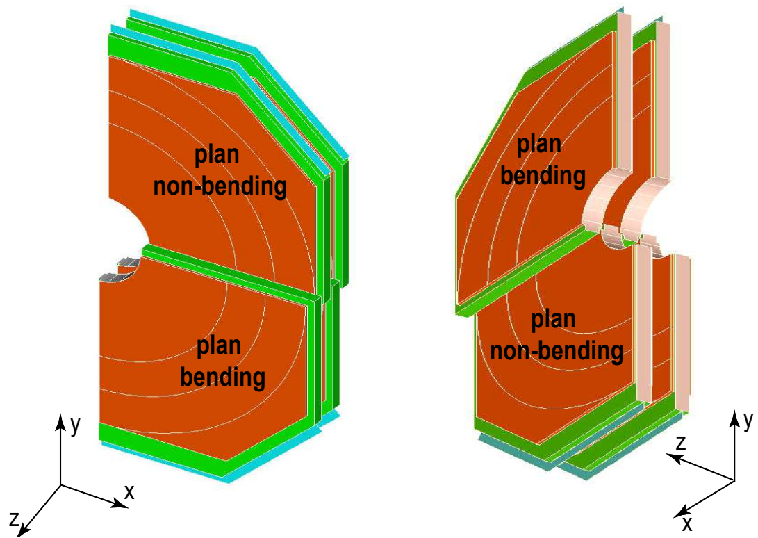
FIG. 4.5 – Disposition de 4 quadrants de la station 1 et 2.
