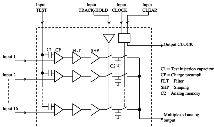
FIG. 4.7 – Design des ASIC MANAS. CP désigne l'opération de pré-amplification de charge, FLT le filtrage du signal et SHP sa mise en forme.
