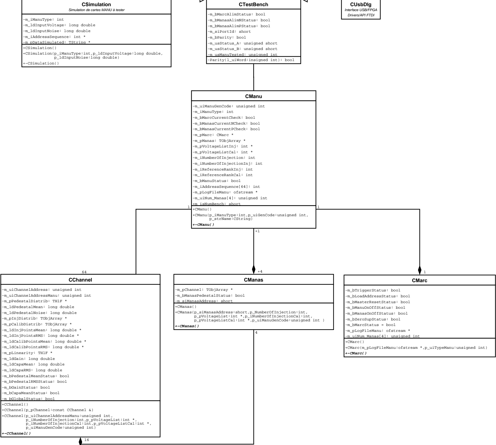
FIG. A.1 – Diagramme UML du logiciel du banc de test industriel. Toutes les classes héritent de la classe de base TObjet de l'environnement ROOT.
