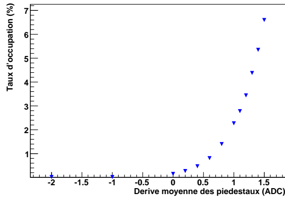
FIG. 6.3 – Evolution du taux d’occupation en fonction de la dérive des piédestaux (en canaux ADC).
