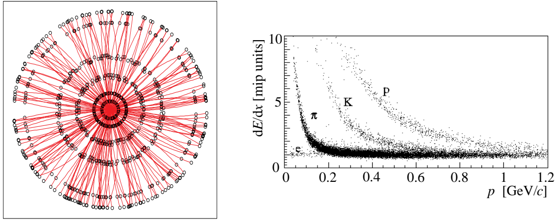
FIG. 3.4 – A gauche : exemple de reconstruction d’un événement dans l’ITS en utilisant les informations fournies par la TPC. A droite : graphe de corrélation entre la perte d’énergie mesurée par l’ITS en fonction de l’impulsion de différentes particules.
