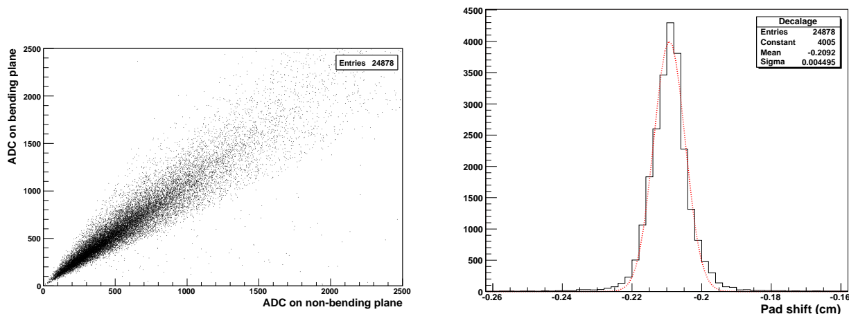
FIG. 5.12 – A gauche : corrélation de charge entre le plan bending (équipé de MANAS) et non-bending (avec GASSPLEX). A droite : décalage des segments de cathode (cm) entre le plan bending et non-bending dans la zone de grande densité de segments. L’histogramme montre la différence de la position du point d’impact calculée sur chaque plan : on y retrouve le décalage des pads entre les deux plans.
