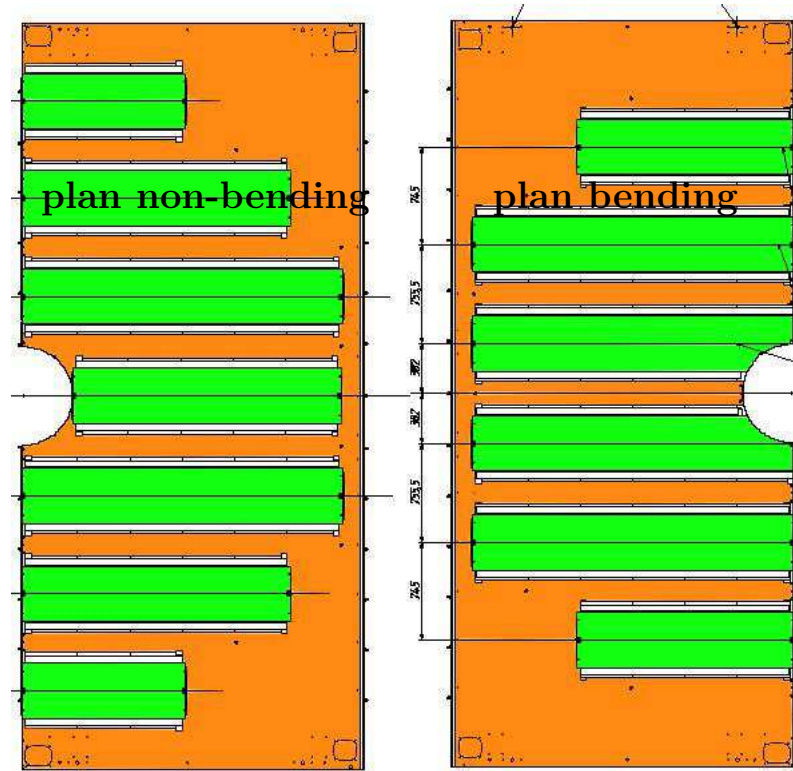
FIG. 4.4 – Vue de face (à gauche) et arrière (à droite) d’une demi-chambre de la station 3 : les lattes sont fixées sur des supports en carbone de manière à recouvrir toute l’acceptance géométrique.
