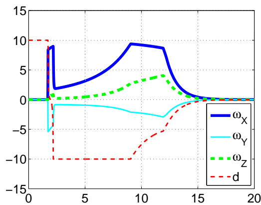
(e) Commande ( m.s^{-1} ou rad.s^{-1} ) en fonction du temps (s)
