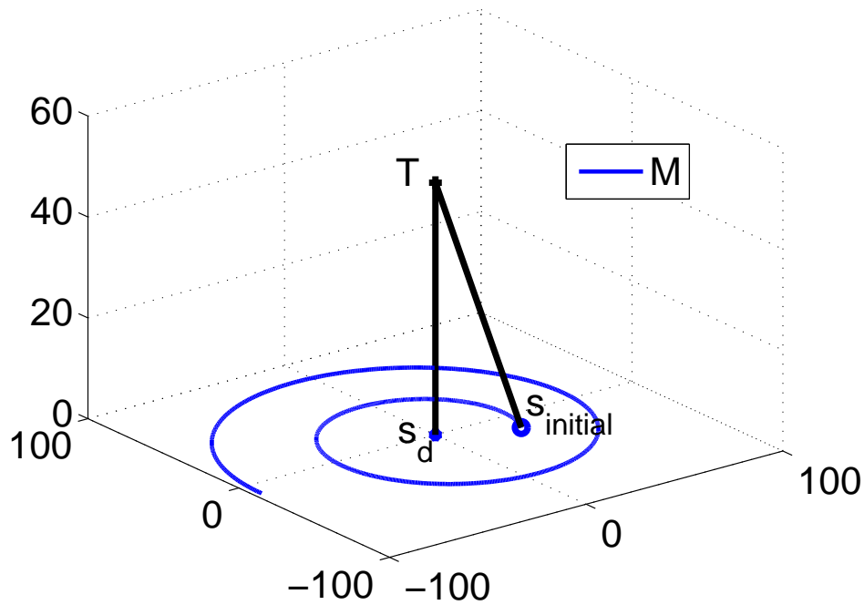
FIG. 2.6 – Résultat (en cm) dans un cas instable : \hat{\theta} = \theta + \pi/2 + 0,1
