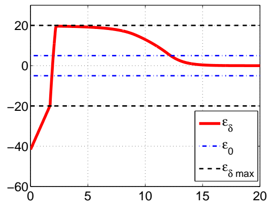
(d) Erreur en \delta (mm) en fonction du temps (s)
