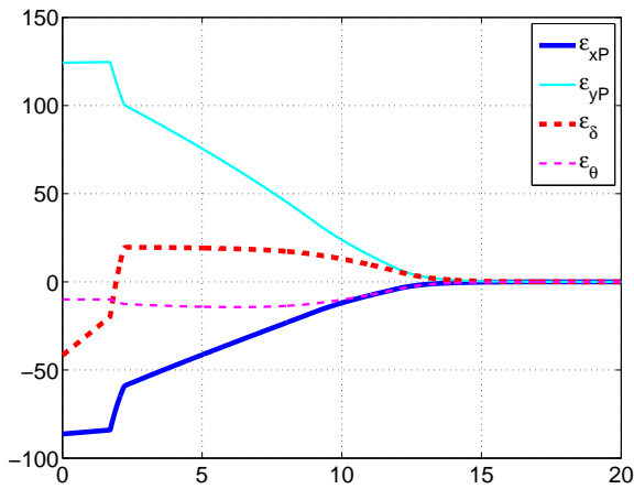
(c) Erreur (m ou rad) en fonction du temps (s)
