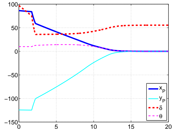
(b) Position courante (m ou rad) en fonction du temps (s)
