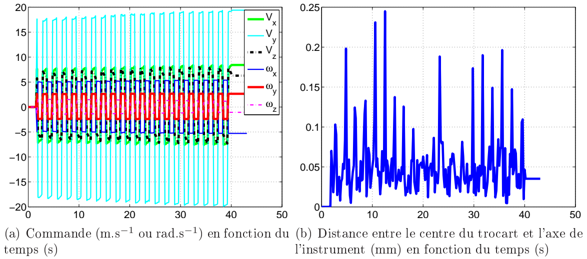
FIG. 3.7 – Correction de la dérive du trocart
