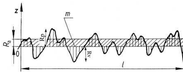
Figure 19. Représentation des paramètres définissant une rugosité de surface. R_a : écart moyen arithmétique du profil, R_p : hauteur de saillie maximale, R_v : profondeur de creux maximal, m : médiane ( http://www.maitrise-orthop.com/corpusmaitri/orthopaedic/mo78_zircone/index_vf.shtml ).
