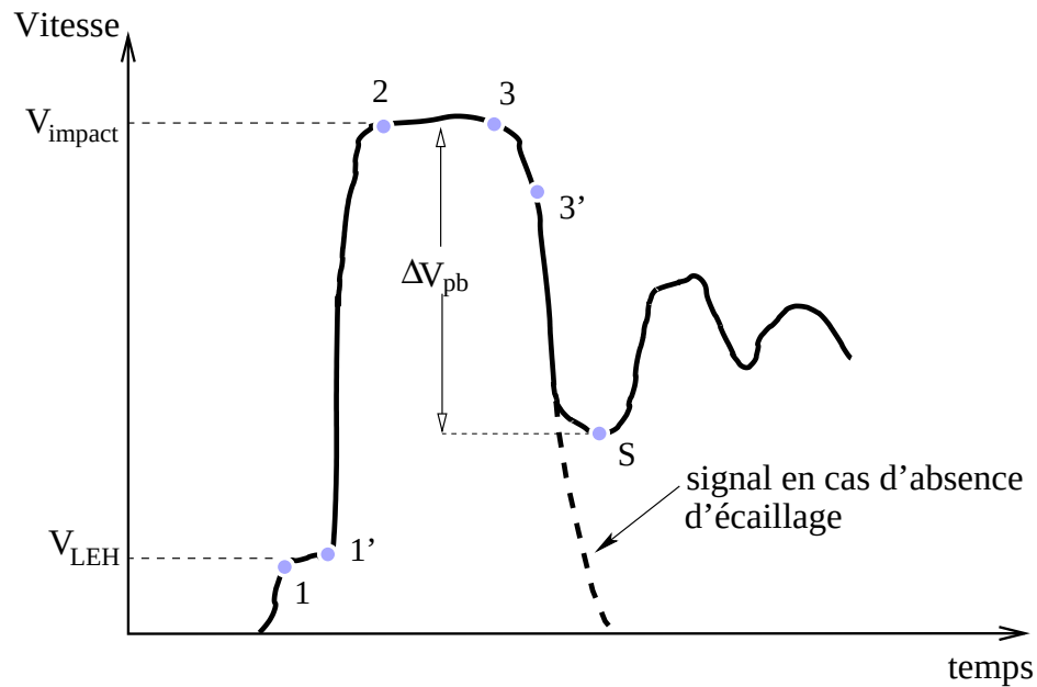
FIG. 4.8 – Vitesse de surface libre type obtenue par un VISAR. Le point S identifie l'apparition de l'écailage au cœur de la cible
