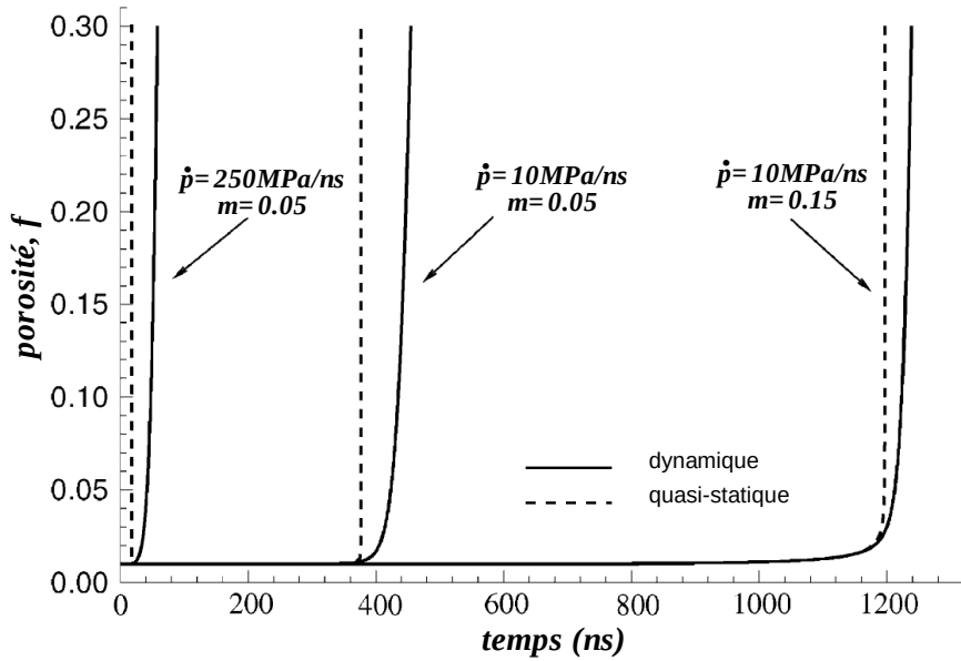
FIG. 2.5 – Expansion dynamique d'un matériau poreux ( \rho = 2700 \text{ kg/m}^3 , A = 245 \text{ USI} , f_0 = 0.1 , a_0 = 20 \mu\text{m} ). Comparaison entre les analyses dynamique (équation (2.69), trait continu) et quasi-statique (équation (2.69) avec \rho = 0 , trait discontinu) pour deux valeurs de sensibilité à la vitesse de déformation ( m = 0.05 et m = 0.15 ) et deux vitesses de chargement ( \dot{p} = 10 \text{ MPa/ns} et \dot{p} = 250 \text{ MPa/ns} ).
