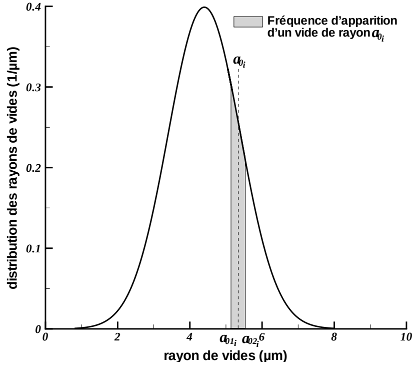
FIG. 2.2 – Distribution de Gauss de tailles initiales de cavités. Les paramètres de la distribution sont donnés dans le tableau 2.1. La fréquence d'apparition d'un motif de rayon initial a_{0i} , représentée par l'aire grisée, est donnée par l'équation (2.6).
