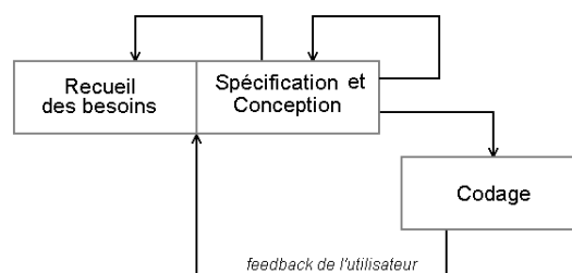
FIG. 3.8 – Modèle par développement évolutif
