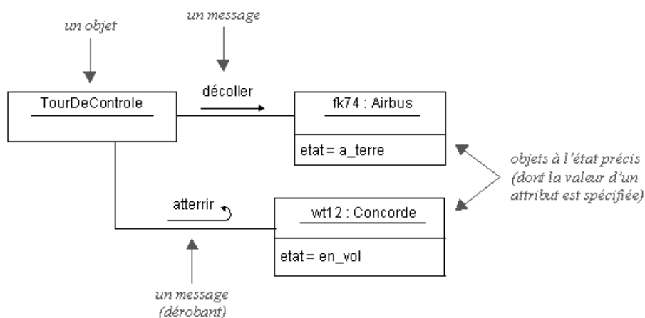
FIG. A.3 – Diagramme de collaboration
