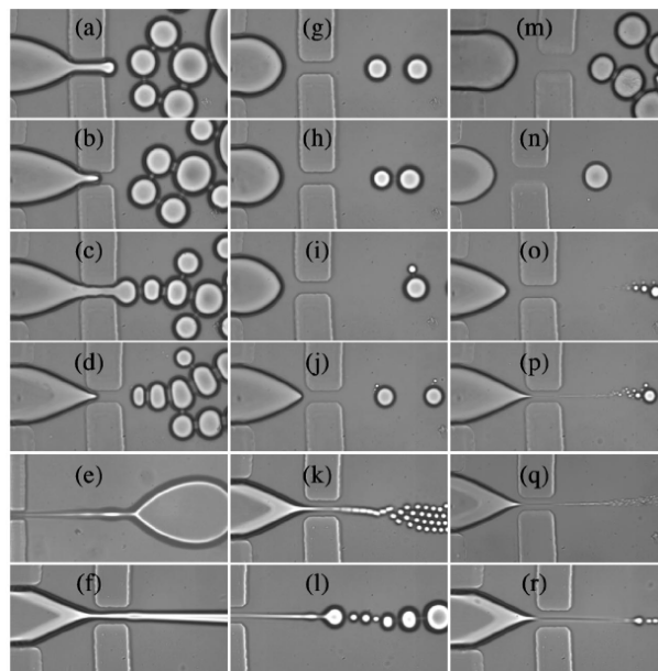
FIG. 7.7 – Différents régimes d'émulsions mis à jour dans [16].
