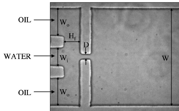
FIG. 7.6 – Configuration "flow focusing" utilisée par Anna et al. dans [16]. Dans le canal central, à gauche, est injectée de l'eau dont le jet se trouve pincé par l'arrivée latérale d'huile. Le mélange bifluide immiscible passe alors au travers du rétrécissement D pour se retrouver dans la cavité de droite (de largeur W ).
