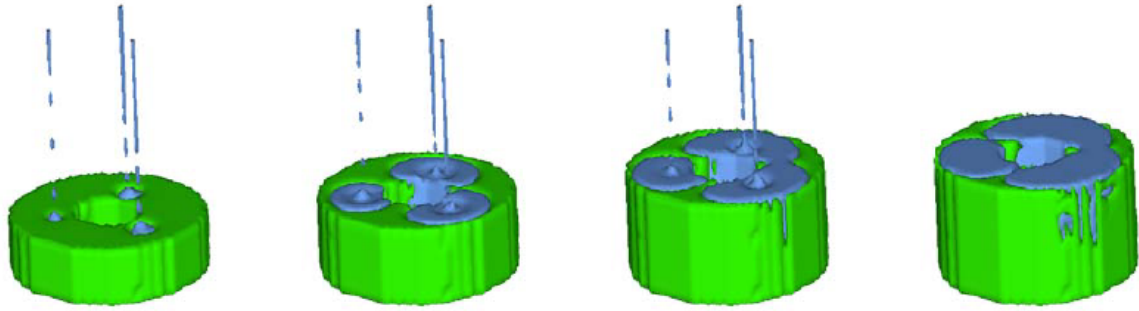
FIG. 1.3 – Simulations de deux coulées successives de propergol dans un booster d’Ariane V [24]. Lors de ce remplissage, qui se fait en une dizaine d’injections à intervalles séparés, le propergol est à l’état liquide mais commence à se solidifier par un processus de réticulation. Il faut prendre garde, lors de ce processus, que des défauts comme des bulles d’air, ne restent pas piégés dans le propergol, une fois qu’il s’est solidifié. En effet, la vitesse de combustion, au décollage de la fusée, en serait altérée.
