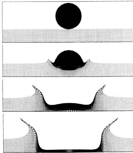
FIG. 1.13 – L'éclaboussure provoquée par l'impact d'une goutte sur une surface libre, simulée par Harlow et Shannon dans un article de 1967 [73] utilisant la méthode MAC
