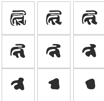
FIG. 1.8 – Illustration du théorème Grayson où une courbe du plan commence à se contracter vers un point, extrait de [147]
