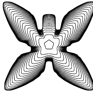
FIG. 1.5 – Simulation en croissance dendritique extraite de [62] : un pentagone (au centre) voit des dendrites se développer préférentiellement suivant les axes diagonaux
