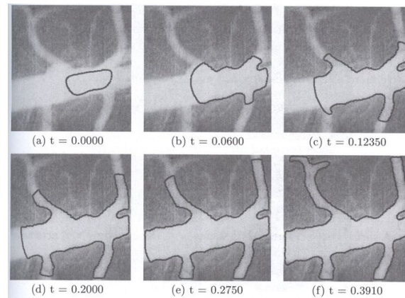
FIG. 1.6 – Une interface (en gris foncé) évoluant pour détecter un réseau artériel en imagerie médicale [104]
