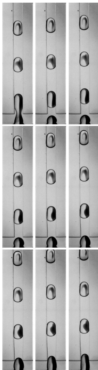
FIG. 8.12 – Quelques instantanés d’une expérience physique [37, 38] où l’on voit des micro-gouttes se former dans un canal en croix et se propager vers le haut. La séquence est ordonnée de gauche à droite puis de haut en bas. Les gouttes contiennent un colorant (couleur foncée, dans la moitié droite) qui se propage essentiellement dans la zone centrale et n’envahit pas l’avant de la goutte, mettant en évidence la zone morte frontale.
