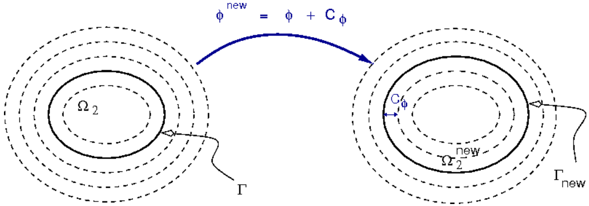
FIG. 5.6 – Méthode de translation pour corriger la variation de masse, selon [157]. Les isovaleurs en gras sont : à gauche, l'ancienne interface et à droite, la nouvelle interface dont l'aire associée vérifie la conservation de la masse.
