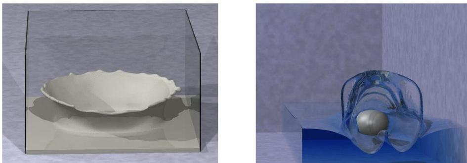
FIG. 2.6 – Simulation Level Set avec des octrees (extraites de [61] et détaillées dans [102]) : à gauche, formation d'un couronne de lait après l'impact d'une sphère ; à droite, une ellipse propulsée juste sous la surface libre. Grâce à cette approche de raffinement du maillage, il est possible de bien capter le développement des films minces, avec des temps de calcul raisonnables.
