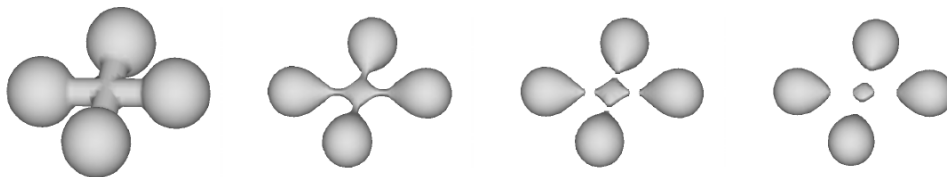
FIG. 1.9 – Illustration du contre-exemple de Grayson où une surface, dans un espace tridimensionnel, se scinde en plusieurs surfaces distinctes, extrait de [35]
