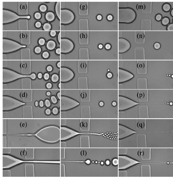
FIG. 7.7 – Différents régimes d'émulsions mis à jour dans [16].
