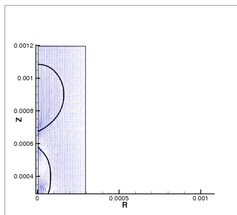
FIG. 9.25 – Développement d'un jet. Temps de référence + 1.6 ms.
