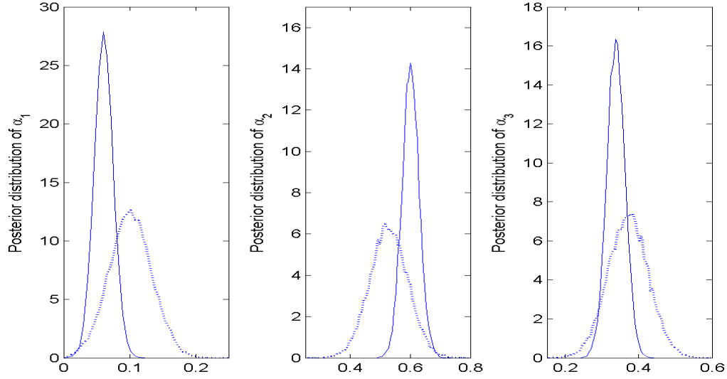
FIG. 3.20 – Lois a posteriori des abondances [\alpha_1, \alpha_2, \alpha_3]^T estimées par l'algorithme proposé (trait plein) et par l'algorithme initial (pointillés).
