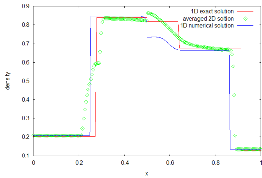
a - densité
