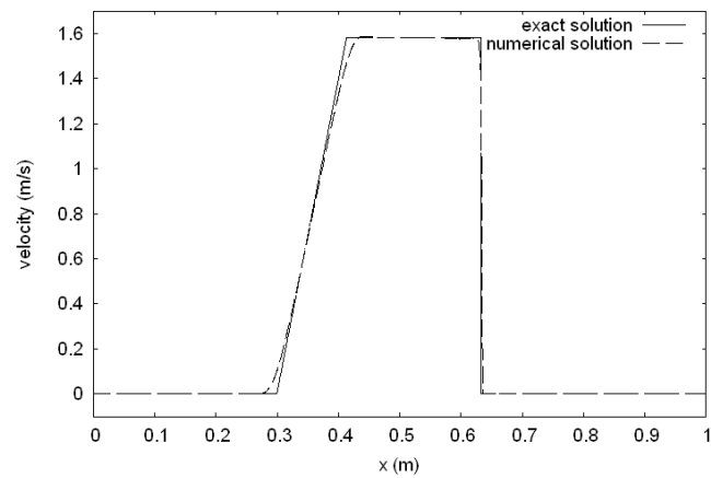
b - vitesse
