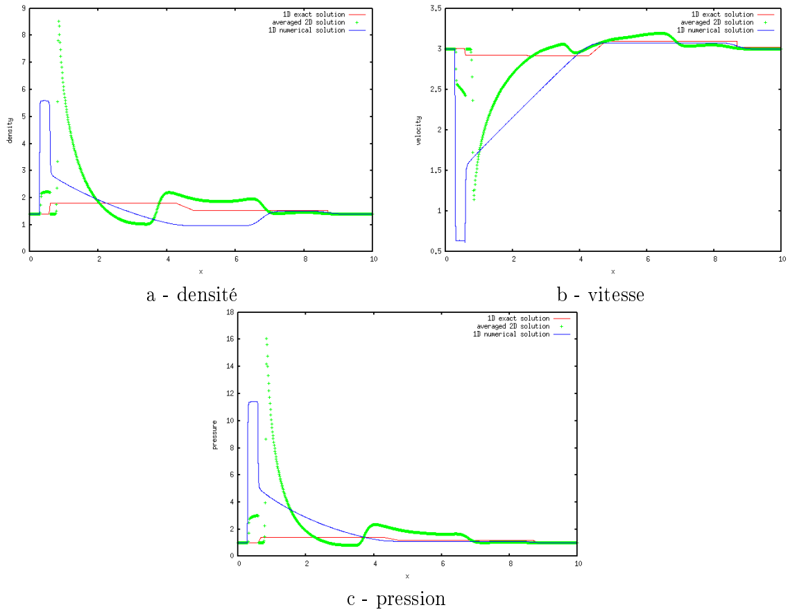
FIG. 3.10 – Solutions du 3 problème de Riemann.
