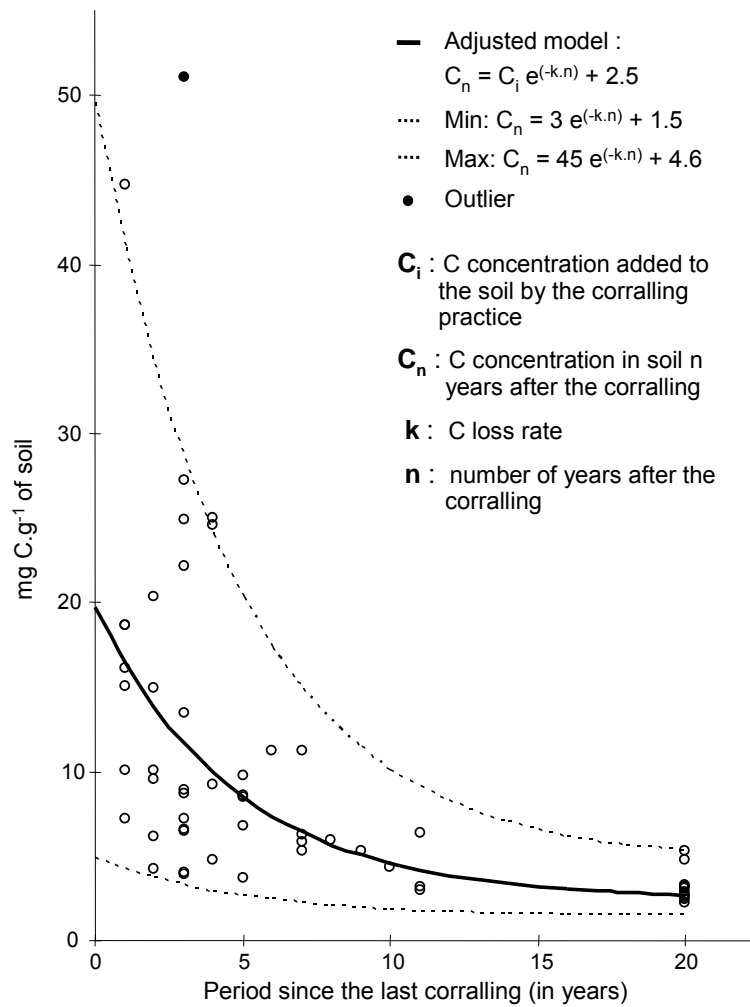
Figure 14 : Teneurs en carbone des sols (0-10 cm) en fonction de la durée après un parage nocturne d'animaux domestiques pendant 2 à 3 mois. Un modèle exponentiel de décroissance de la relation entre teneur en carbone et durée après parage a été ajusté.
