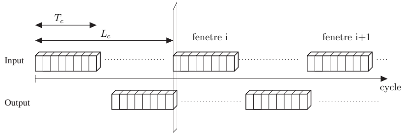
FIG. 3.9 – Illustration du séquençage sériel. Une fenêtre de décodage peut commencer à être traitée quand le résultat du décodage de la précédente est disponible.
